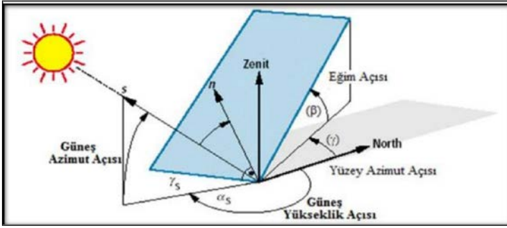
Şekil 3. Güneş açıları
