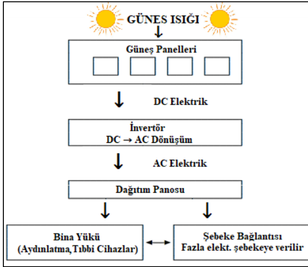
Şekil 2. Fotovoltaiik sistem şeması
