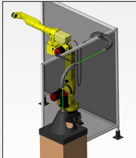
安装在工作站
