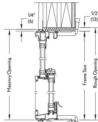
Jamb
