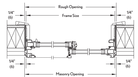
Jambs
