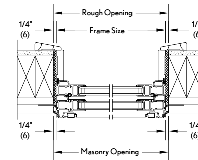
Jamb
