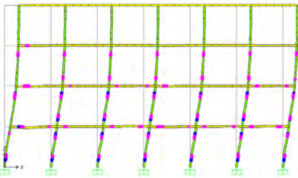
Modelo de pórtico equivalente con plasticidad concentrada y curvas de capacidad.
