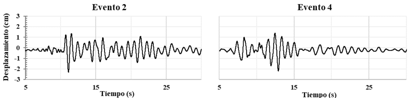
Historia del desplazamiento en el último nivel, dirección longitudinal (L) del edificio para los eventos sísmicos 2 y 4. Sismo 1967.
