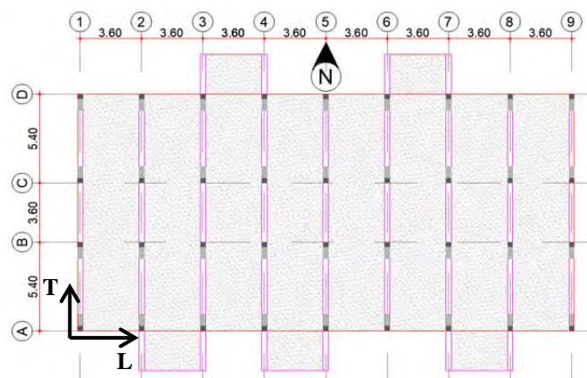
Edificio Belaire. La dirección transversal T (fuerte) del edificio corresponde a la dirección N-S.
