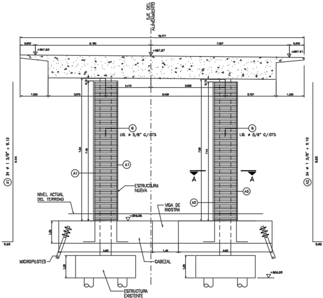
Imagen extraída de los planos de ingeniería de detalle del refuerzo. Engrosamiento de las columnas y nuevas fundaciones. Elevación transversal de una pila con las columnas reforzadas y el cabezal con micro-pilotes inclinados
