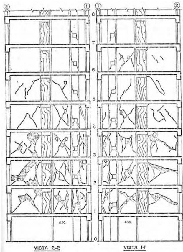
Edificio Petunia I. Izquierda: representación de daños en paredes transversales (adaptado de Arcia & Malaver, 1974); Figura 7.10 derecha: daños en paredes de fachada (Steinbrugge, 1967)
