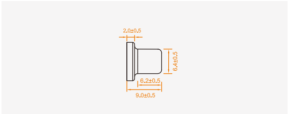
Integral end cap
