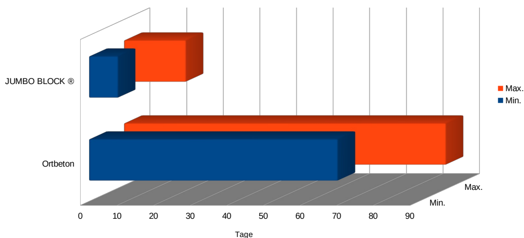
BAUZEIT ORTBETON VS JUMBO BLOCK ® Vergleichbarer Speicher 1362 m 3 / 98 JUMBO BLOCK ®
