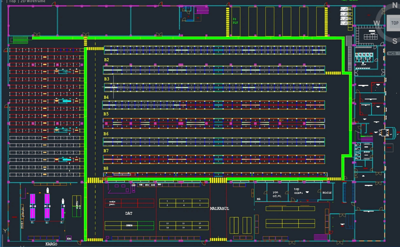
Layout planı
