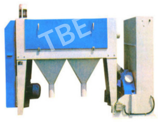
HORIZONTAL SCOURER
