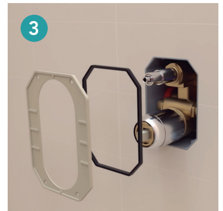
3 Colocar la junta y el protector. Fit the joint and the protector. Situier le joint et le protecteur. Coloque a junta e o protetor.
