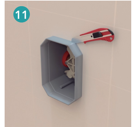
11 Realizar el corte del perfil sobrante de la caja iClever. Instalación de la caja iClever finalizada. Cut the excess profile of the iClever box. Installation of iClever box completed. Couper la partie excédentaire du profil du boîtier iClever. L'installation de l'iClever est terminée. Corte o perfil em excesso da caixa de iClever. Instalação da caixa iClever concluída.
