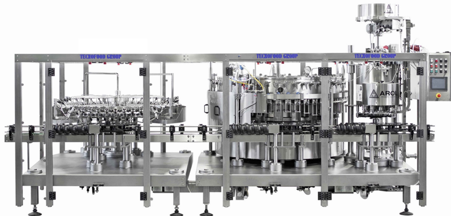
Триблок мод. "TFG S 40/44/8 PK"
