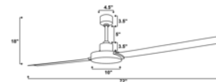
Size Chart Helios 2-Blade Fan
