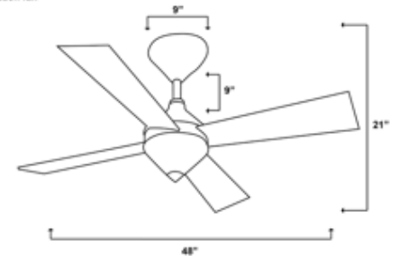
Size Chart Eden fan
