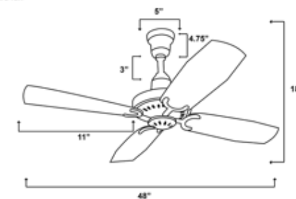
Size Chart Era fan
