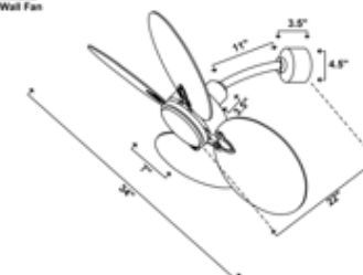
Size Chart Bacca Wall Fan
