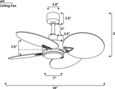
Size Chart Bacca Ceiling Fan
