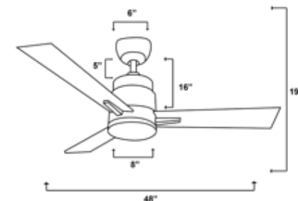
Size Chart Desire fan
