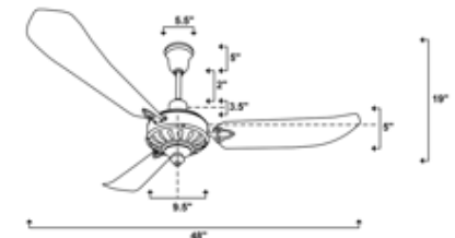
Size Chart Majestic 1945 Fan
