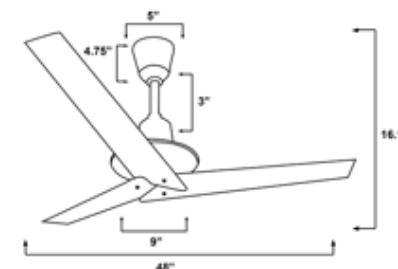
Size Chart Florence fan
