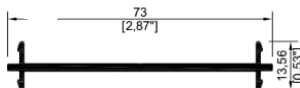
10266 Moldura union 3"
