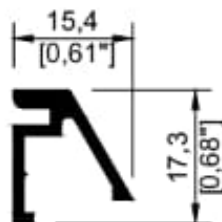
6371 Junquillo biselado
