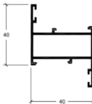
4034 Hoja ventana
