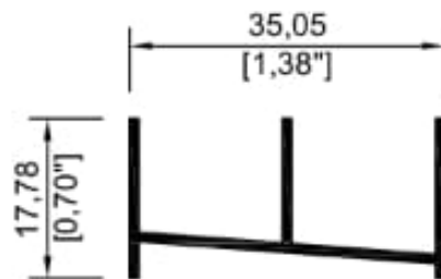
9945 Riel inferior economico
