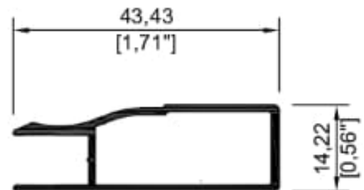
9756 Marco semilujo
