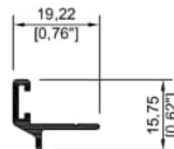
10220 Adaptador oxo
