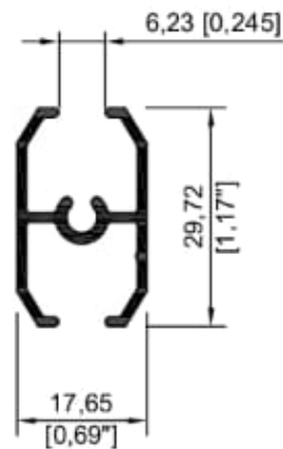
22129 Cuadricula
