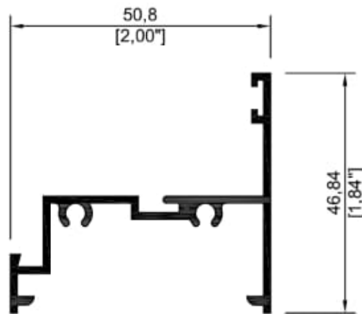
8937 Contra marco
