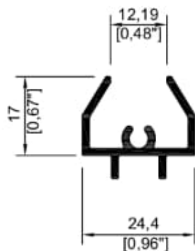
4702 Recercado 3"
