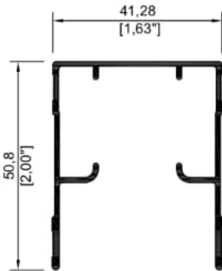
11174 Riel superior economico
