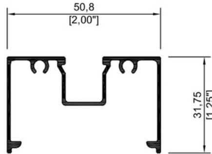
9083 Bolsa 2"
