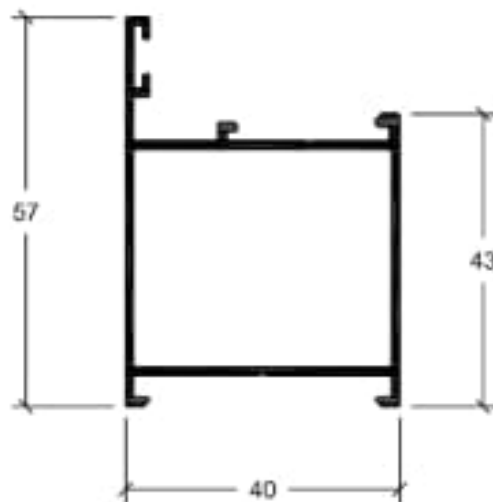
4036 Cerco puerta
