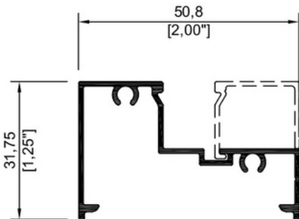
9084 Escalonado 2"
