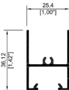
7836 Cabezal 3"
