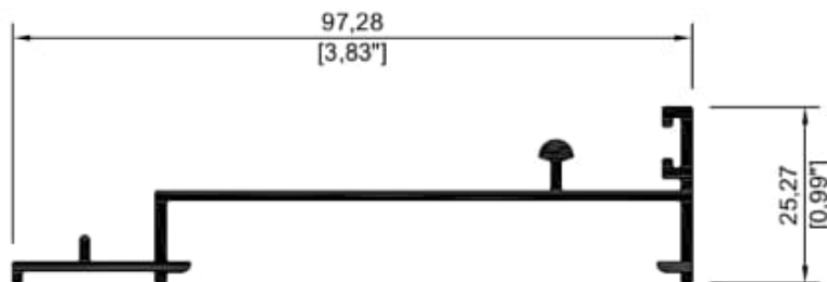
9272 Riel mosquitero 3"
