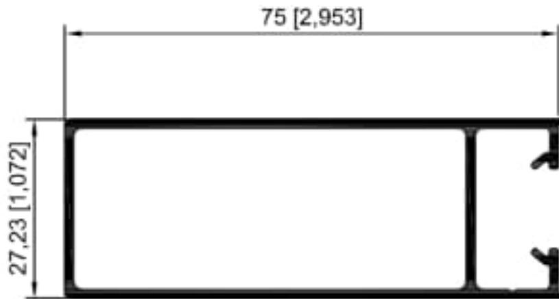
7867 Cerco 3" residencial
