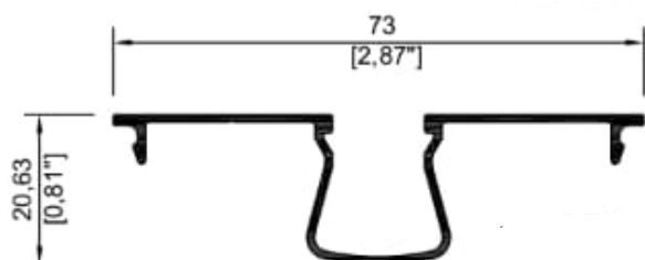
7315 Tapa bolsa 3"
