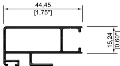
9955 Traslape 2"
