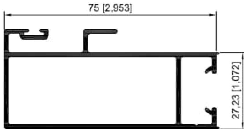
7868 Traslape 3" residencial
