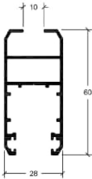
7536 Hoja perimetral 6mm
