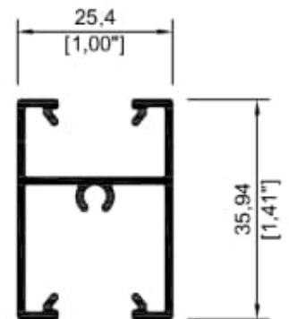
9082 Intermedio 3"
