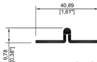
7828 Riel adaptador 3"
