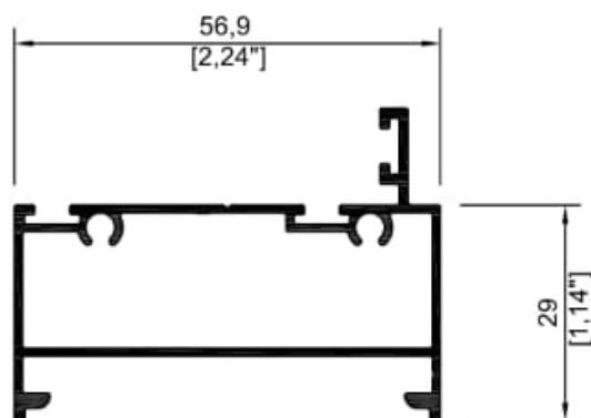
4401 Batiente
