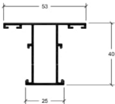
4035 Pilastra ventana
