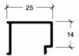
4011 Junquillo 6mm
