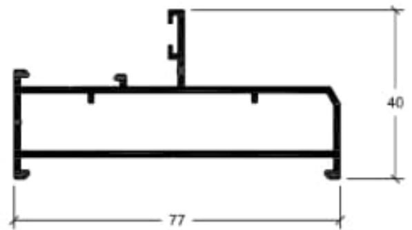
7514 Cerco fijo perimetral
