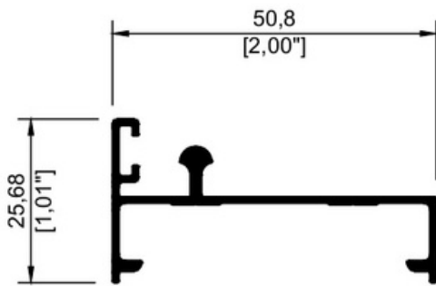
9953 Riel 2"
