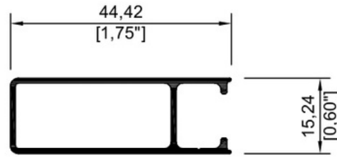
7821 Cerco 2"
