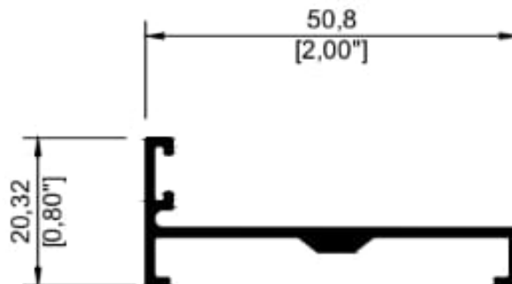
5844 Batiente
