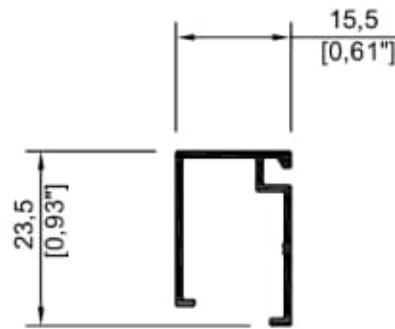
4405 Junquillo recto
