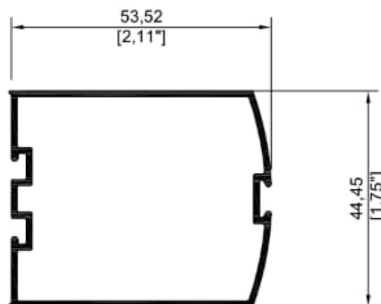
9204 Cerco
