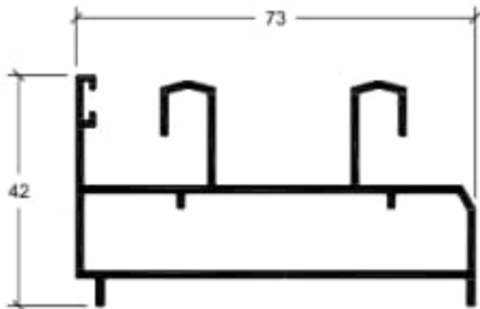
7533 Cerco perimetral
