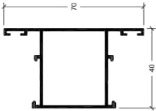
4038 Pilastra puerta
