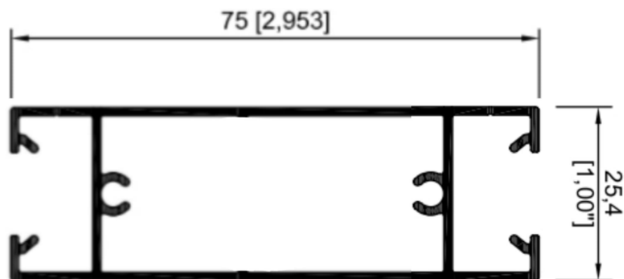
24079 Intermedio 3" residencial
