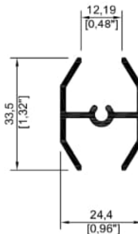
4918 Cuadricula
