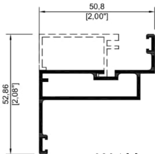
8936 Marco tubular
