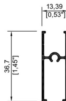
11044 Cabezal 2"
