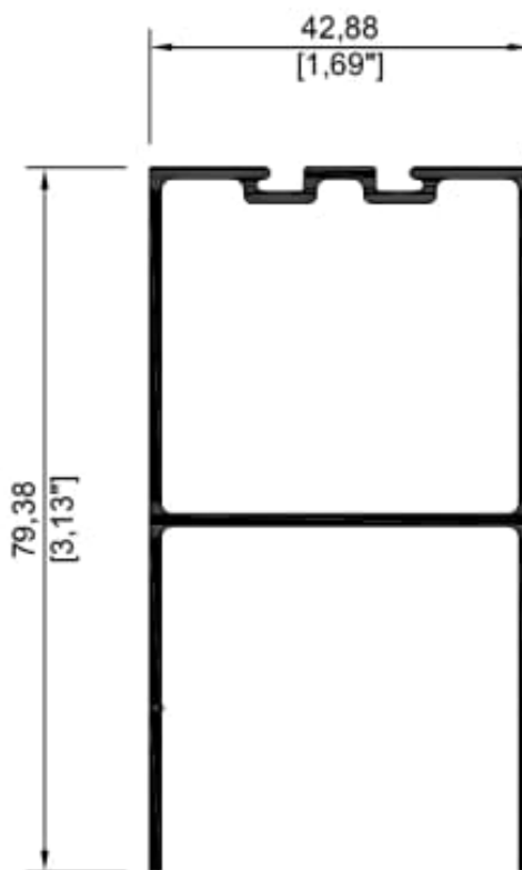
9187 Zoclo
