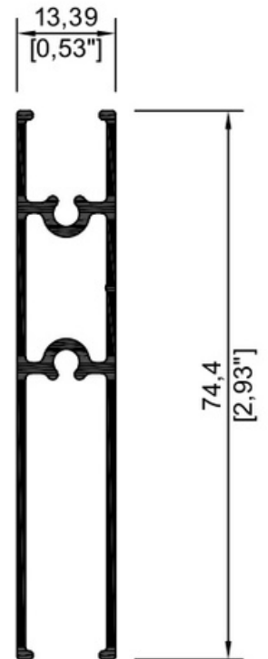
7825 Zoclo 2"
