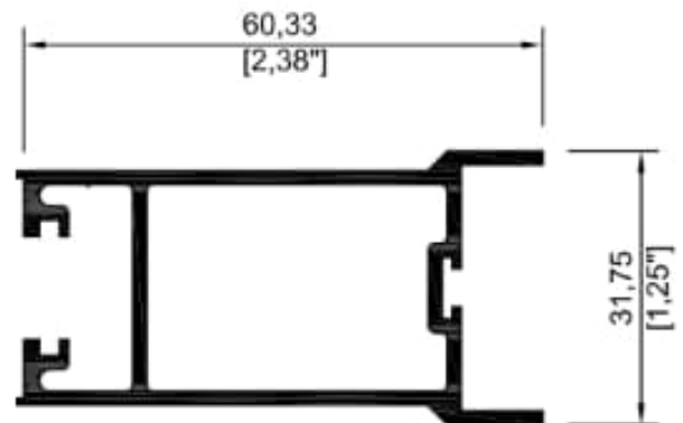
7850 Cerco oxo 3"
