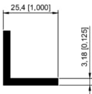
1308 Angulo 1" P/escuadra
