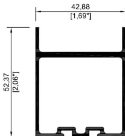
9207 Cabezal
