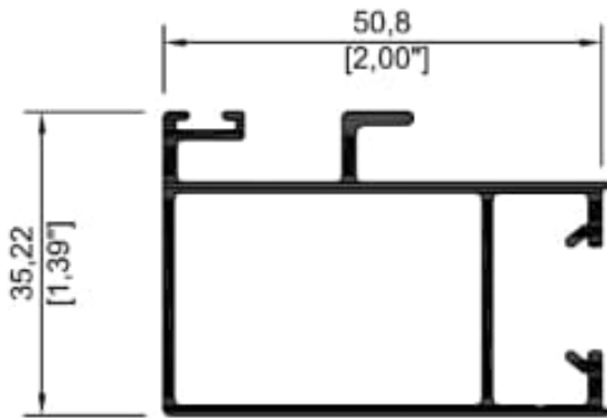
7848 Traslape 3"
