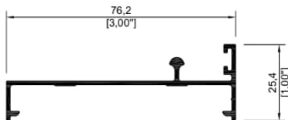
9957 Riel 3"
