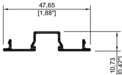
9085 Tapa bolsa 2"
