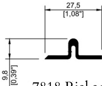
7818 Riel adaptador 2"
