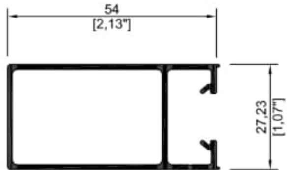
9236 Cerco chapa puerta
