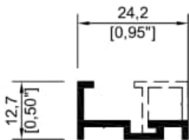
7013 Base portavidrio
