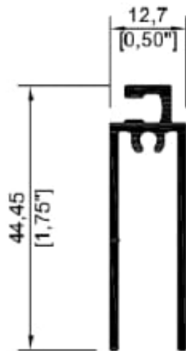
6533 Mosquitero horizontal
