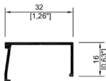
9112 Junquillo 3"
