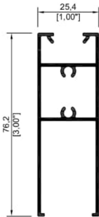
7842 Zoclo puerta 3"
