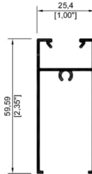
7835 Zoclo 3"
