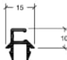
7510 Adaptador moquitero
