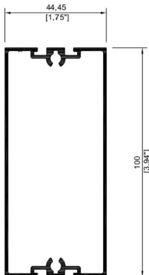
4404 Intermedio
