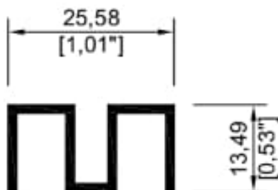
3329 Guia vitrina
