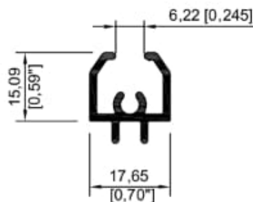
22132 Recercado
