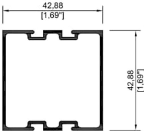
9183 Intermedio
