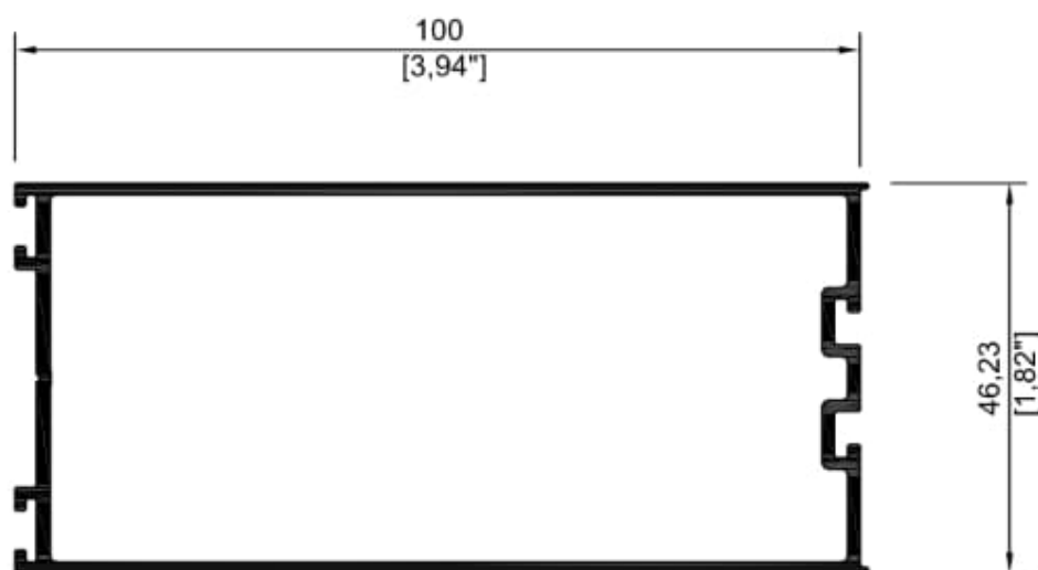
4402 Cerco
