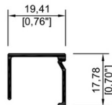
9088 Junquillo 2"
