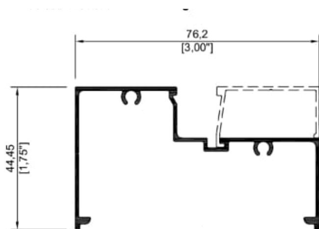
9136 Escalonado 3"
