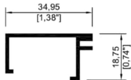
8939 Junquillo
