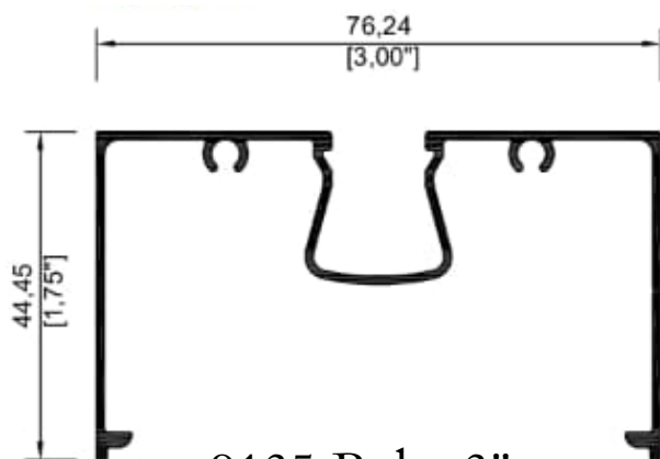
9135 Bolsa 3"
