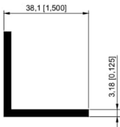
14 Angulo 1 1/2" P/escuadra
