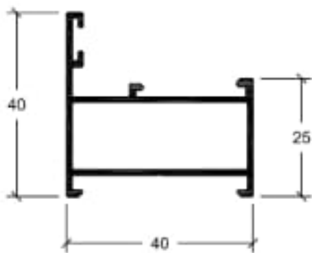
4031 Cerco ventana
