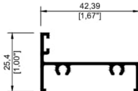
8550 Batiente con venas
