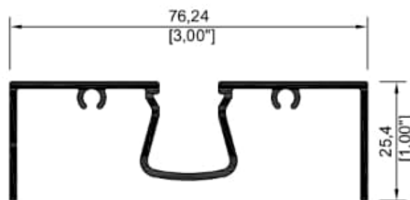
10235 Bolsa corta 3"
