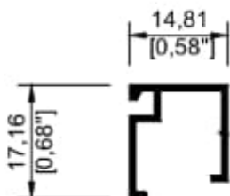
6370 Junquillo
