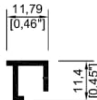
7014 Junquillo portavidrio
