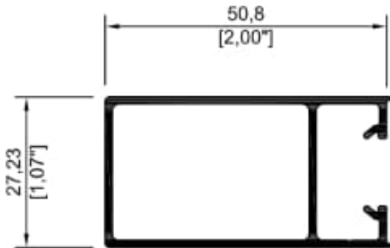
7847 Cerco 3"
