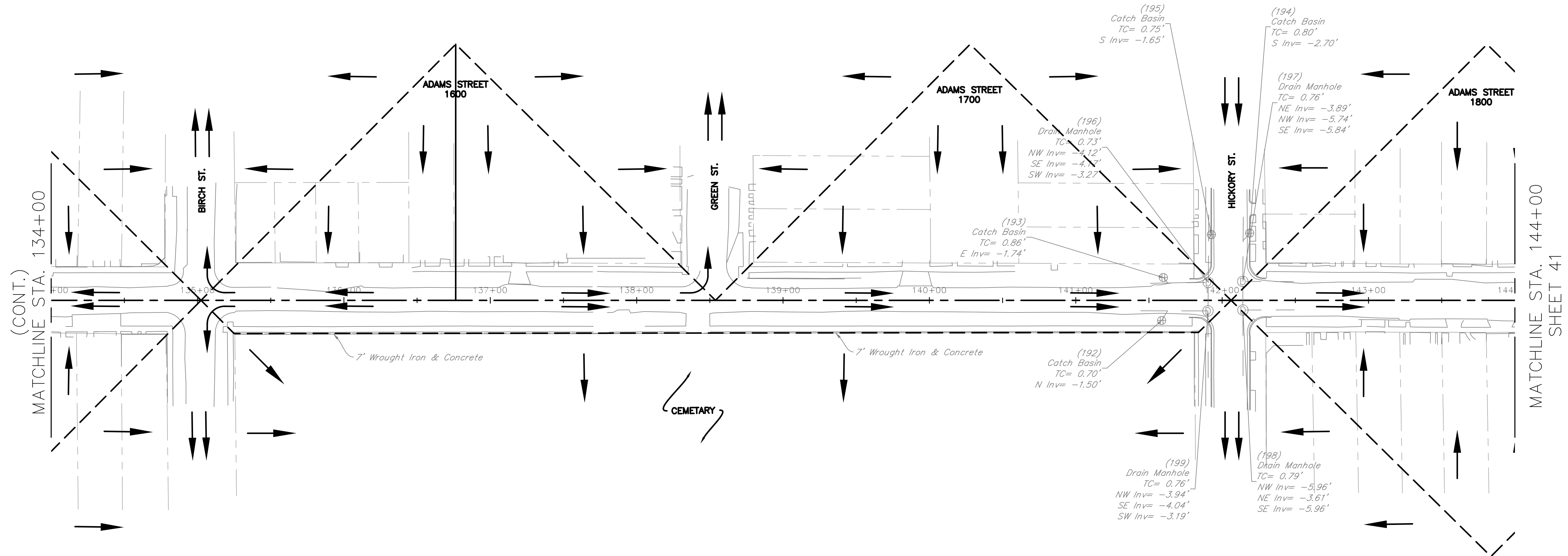
EXISTING DRAINAGE MAP: ADAMS STREET (STA. 134+00 THRU STA. 144+00)
