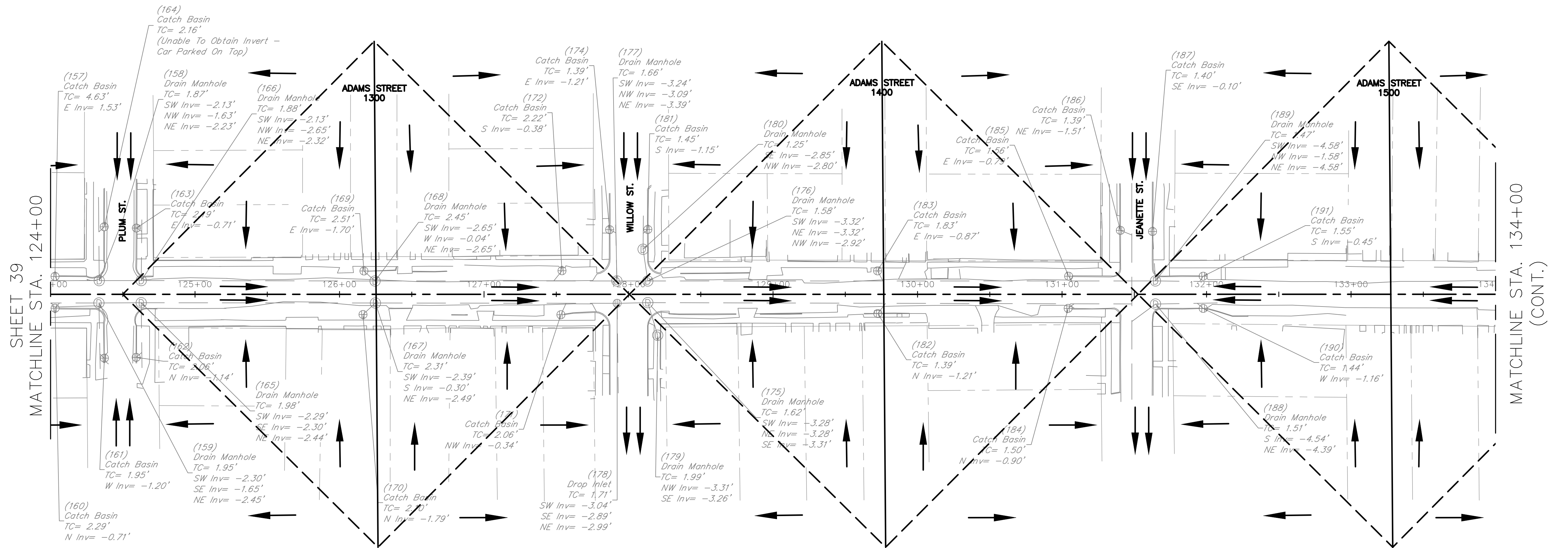
EXISTING DRAINAGE MAP: ADAMS STREET (STA. 124+00 THRU STA. 134+00)
