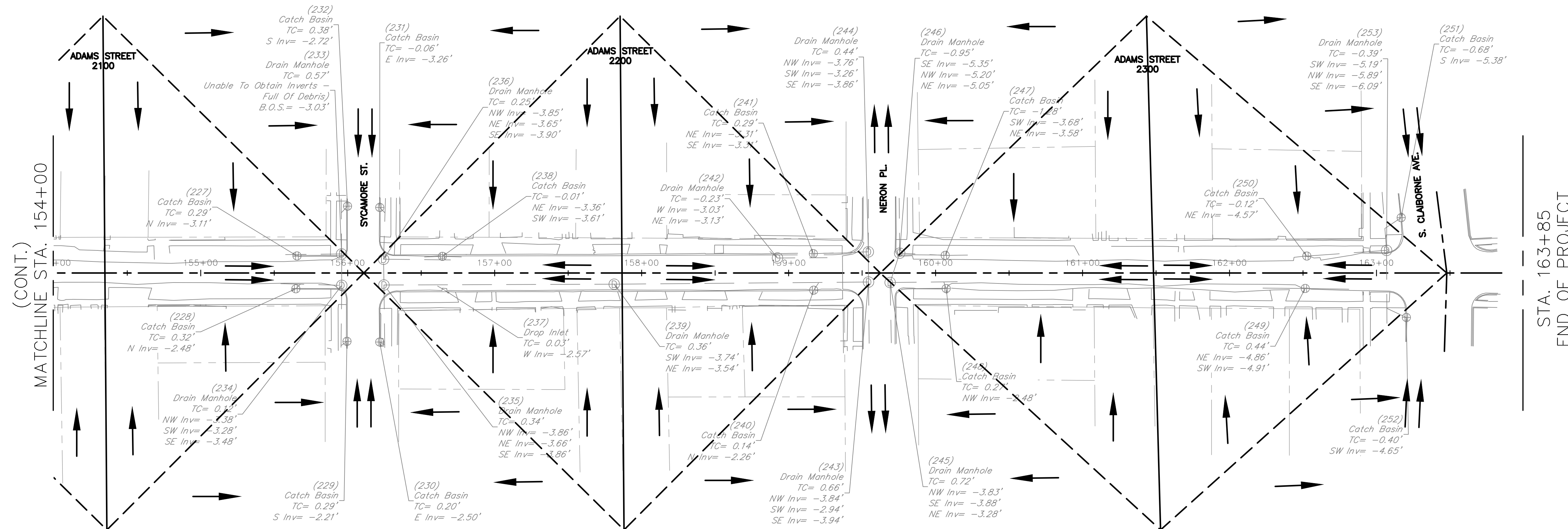
EXISTING DRAINAGE MAP: ADAMS STREET (STA. 154+00 THRU STA. 163+85)
