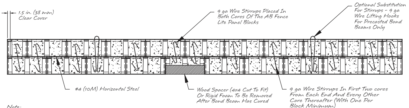
Longitudinal Cross Section
