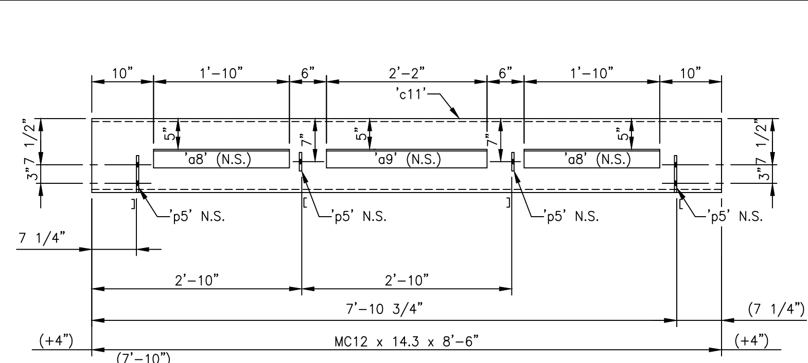
'14B1' ASSEMBLY SCALE: N.T.S.
