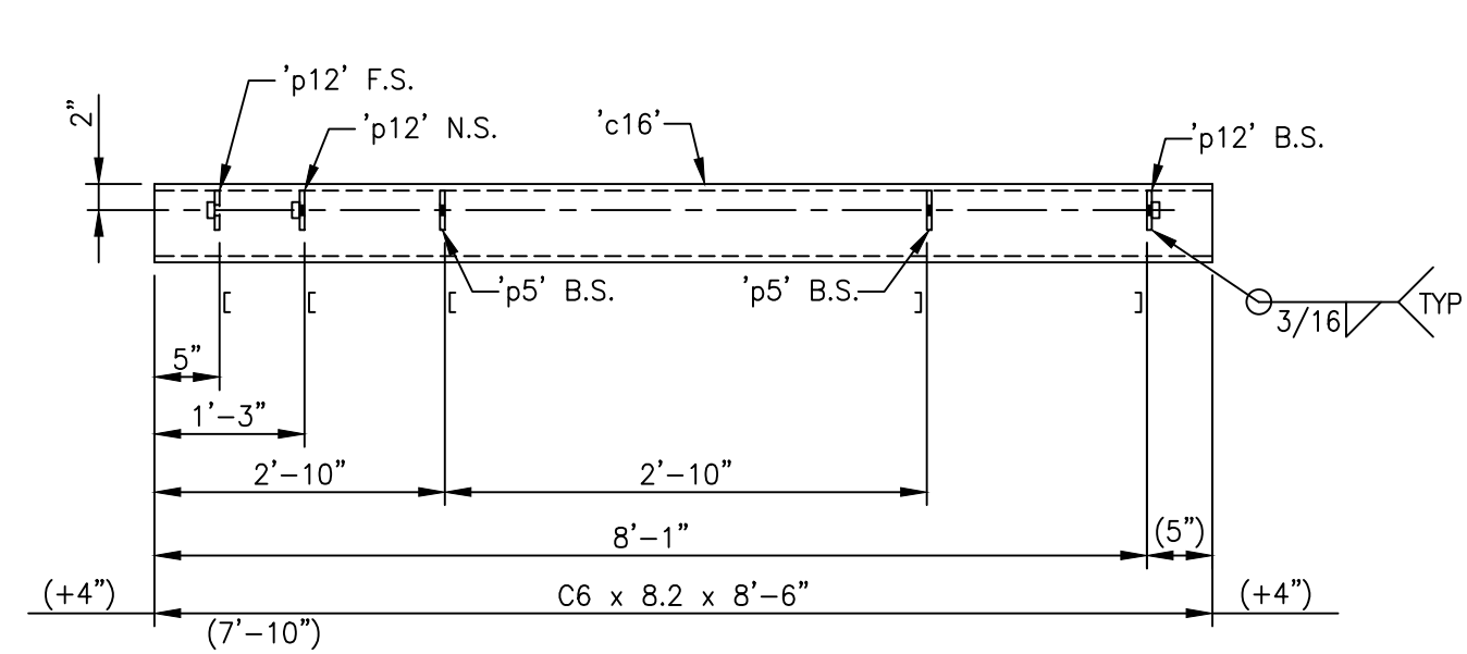
'14B7' ASSEMBLY SCALE: N.T.S.
