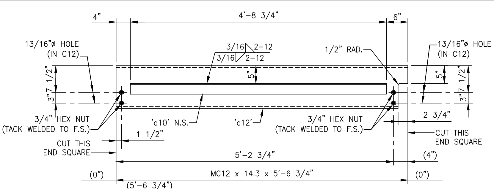
'14B2' ASSEMBLY (AS SHOWN) SCALE: N.T.S. '14B3' ASSEMBLY (OPP HAND) SCALE: N.T.S.
