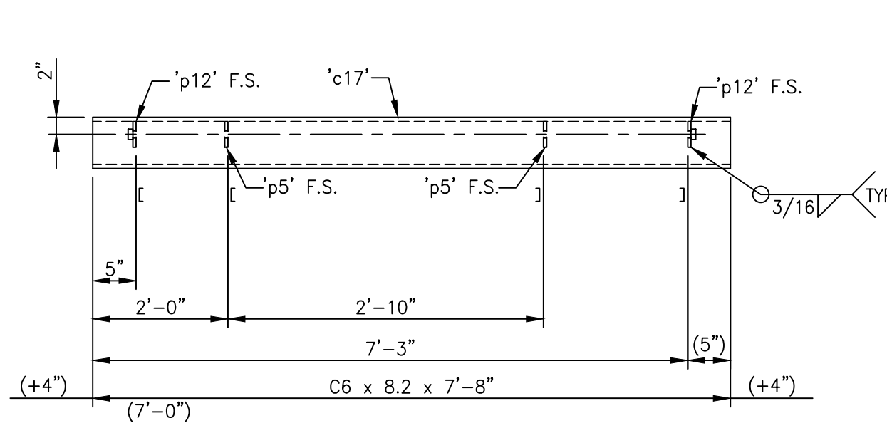
'14B8' ASSEMBLY SCALE: N.T.S.
