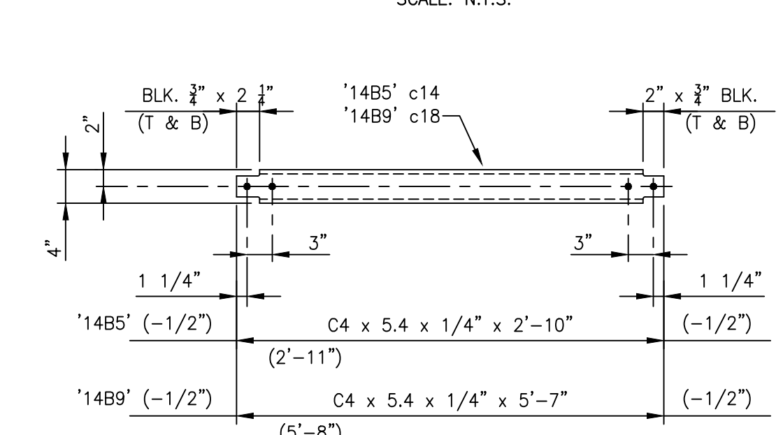
'14B5' ASSEMBLY SCALE: N.T.S. '14B9' ASSEMBLY SCALE: N.T.S.
