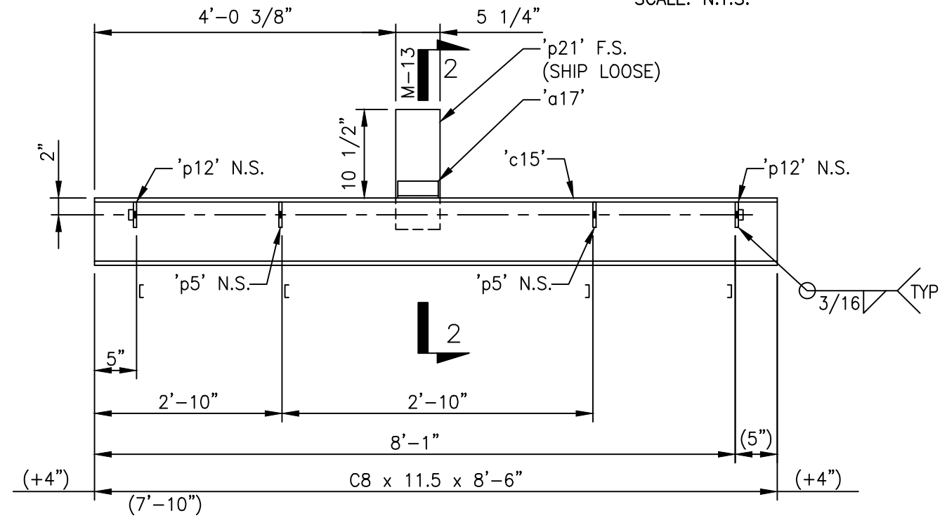
'14B6' ASSEMBLY SCALE: N.T.S.
