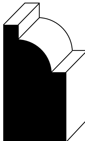
SDW703 1-1/16" x 2"
