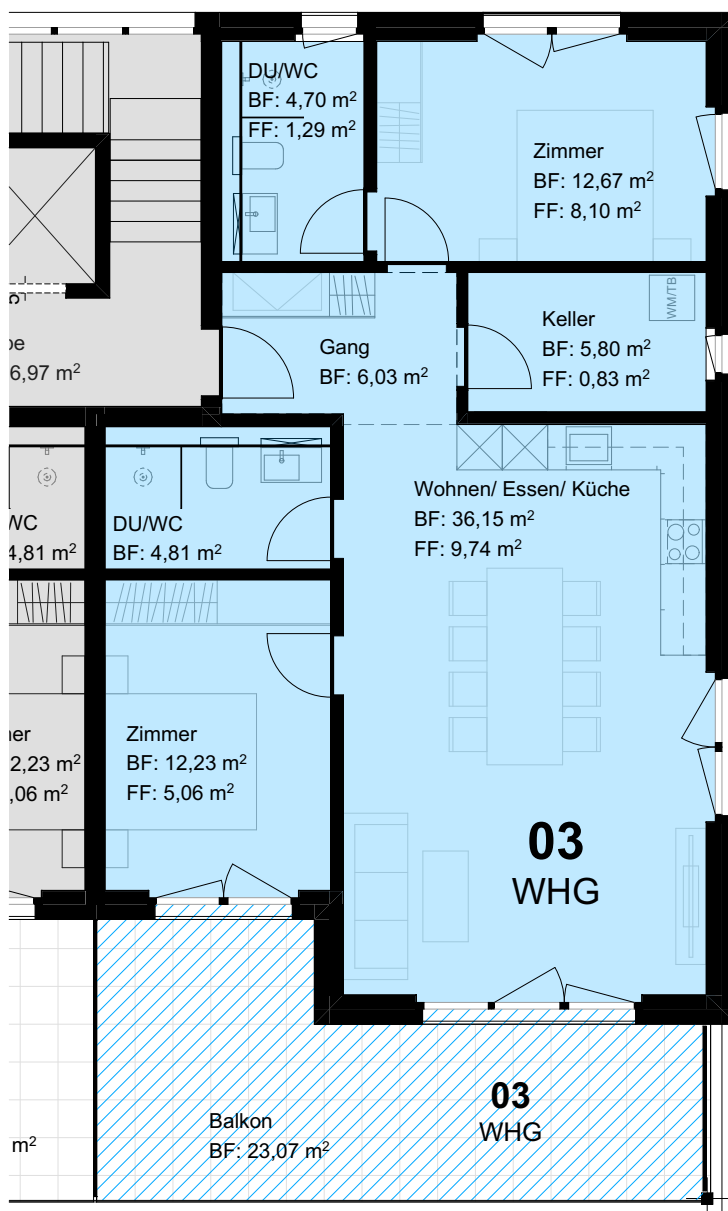
1.OG Wohnung 3
