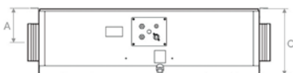
Vista lateral
