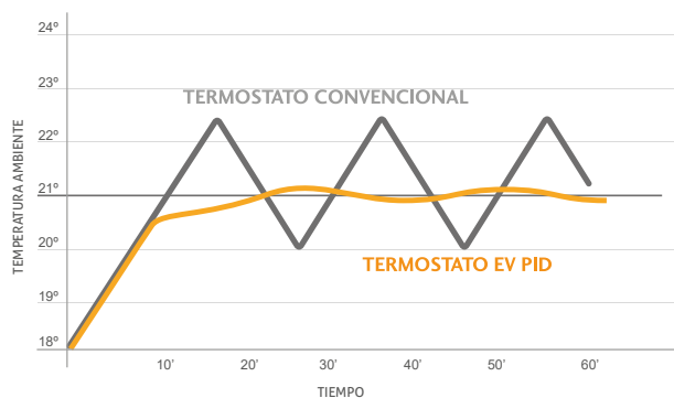
Gráfico comparativo de las variaciones de temperatura con consigna de 21^{\circ}\text{C} .
