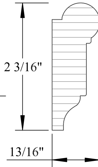
R0-023
