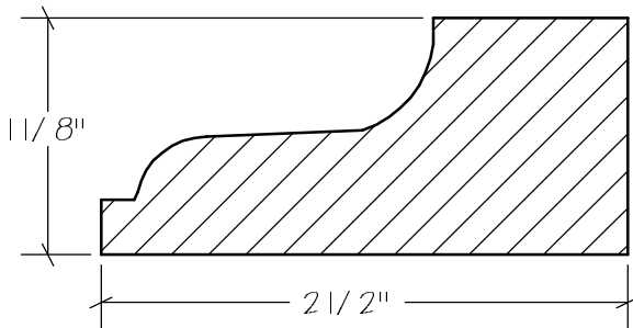
Q0-012
