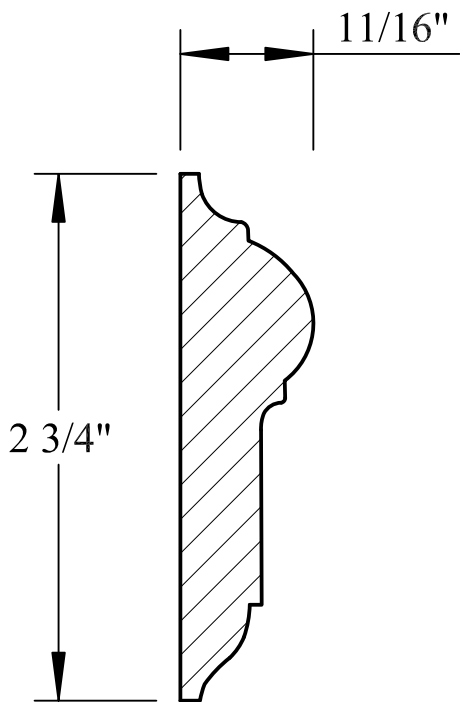
M0-067
