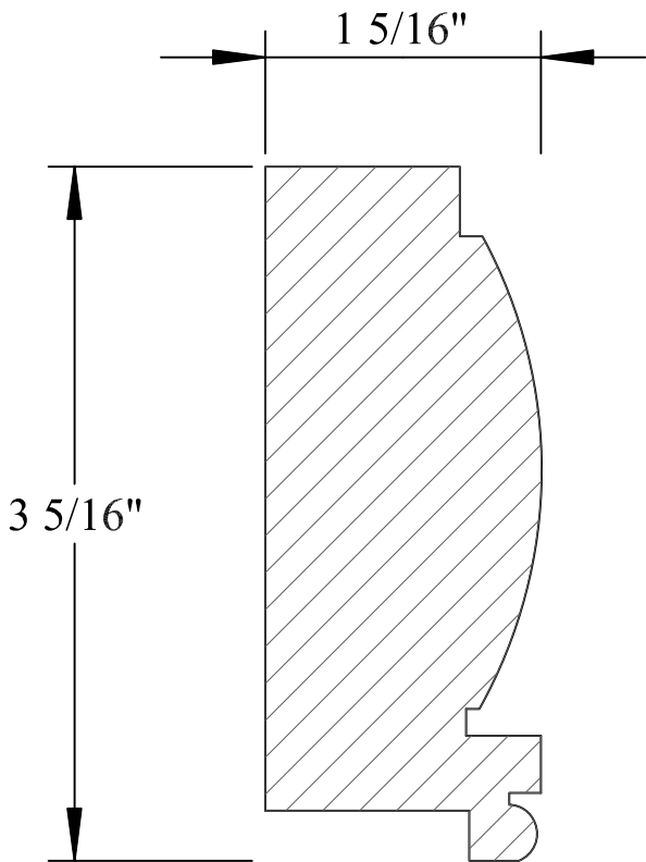
M0-121
