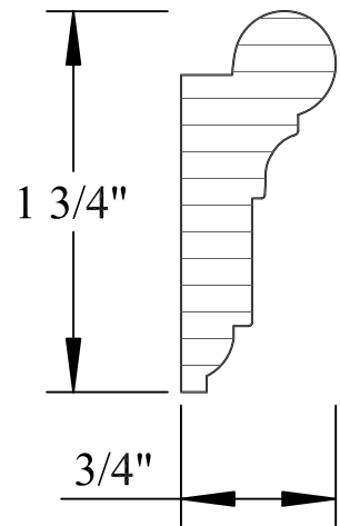
R0-020
