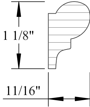
R0-018
