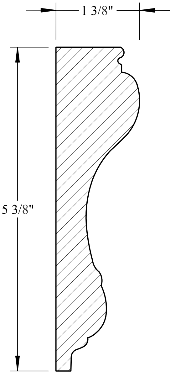
M0-068
