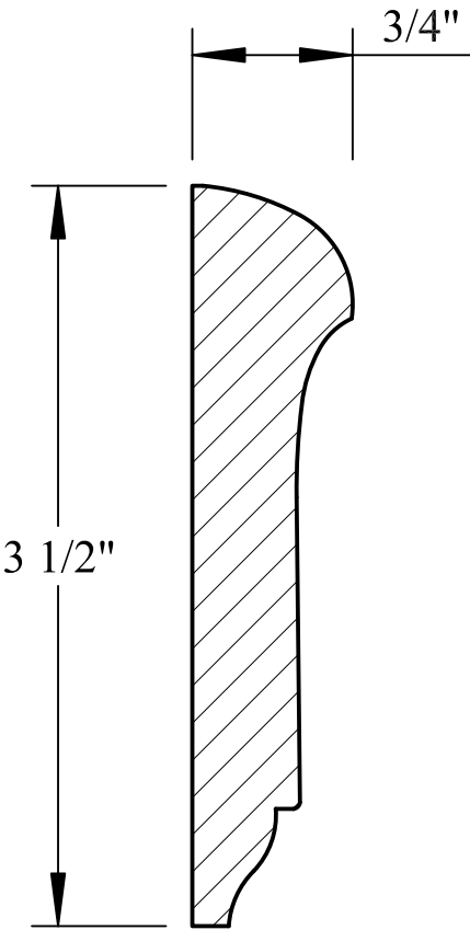
M0-085
