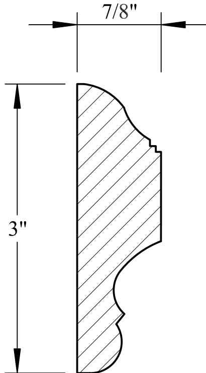
M0-090
