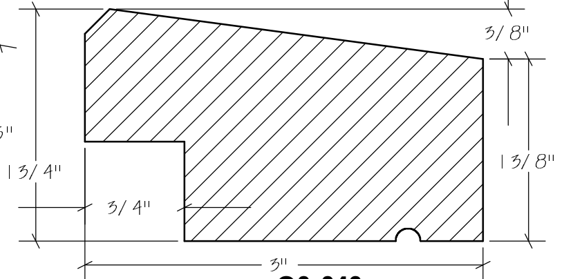
Q0-046
