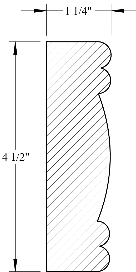
M0-088
