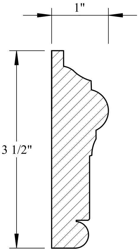
M0-066
