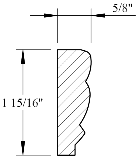
M0-065
