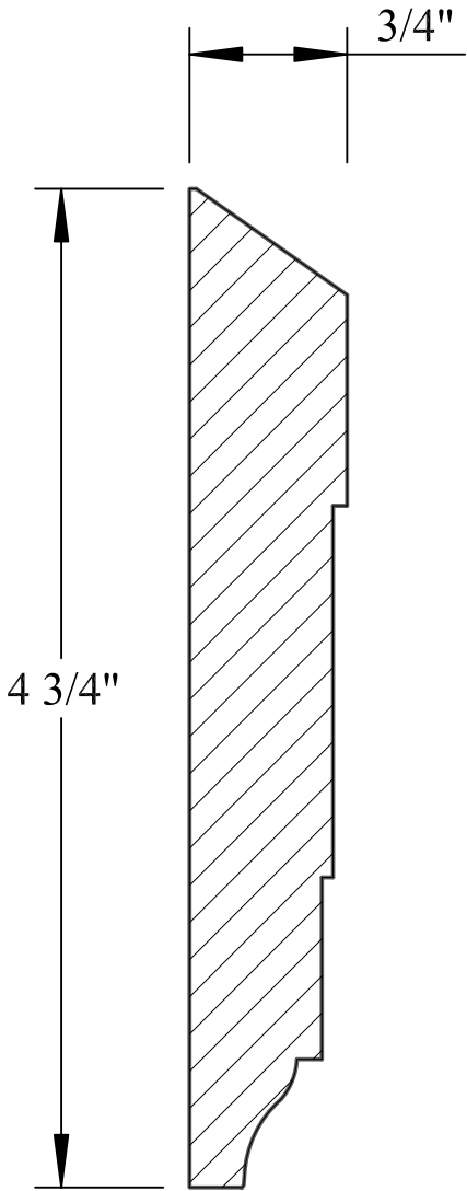
M0-087
