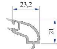
24 mm Dekoratif Contalı Çift Cam Çıtası P.A.750.4204.600.0.HC
