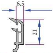
42mm Contalı Üçlü Cam Çıtası P.A.532.4500.600.0.HC
