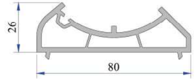
Açılı Köşe Dönüş Adaptörü P.A.080.5104.600.0.00.19
