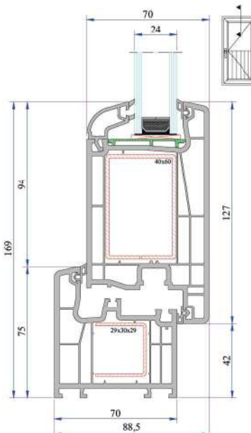
Kasa - Dışa Açılım Süper Kapı Kanat Montajı
