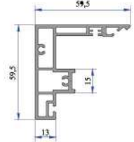
Alum. Sürme Orta Kayıt 3 Odacıklı (Yeni Yapılacak)
