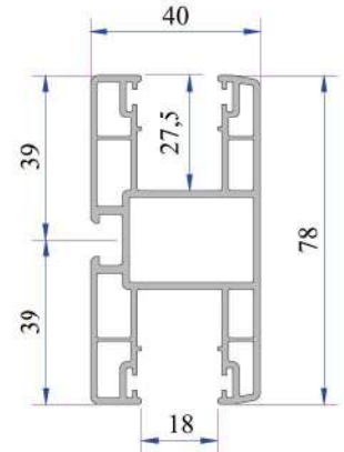
55'lik Lamel Orta Ray P.A.097.5614.600.0.00.19
