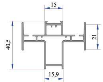
Alm. Kulaklı Çift kanat Ara Adaptörü (Profil Yeni Yapılacak) AD16-058
