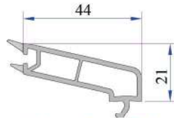
4-6 mm Contalı Tek Cam Çıtası P.A.750.4000.600.0.HC
