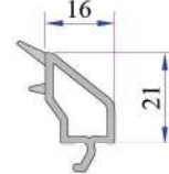
Contalı Çift Cam Çıtası 24 mm 750.4500
