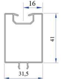
Panjur Yan Ray Yükseltme Profili AD16-050
