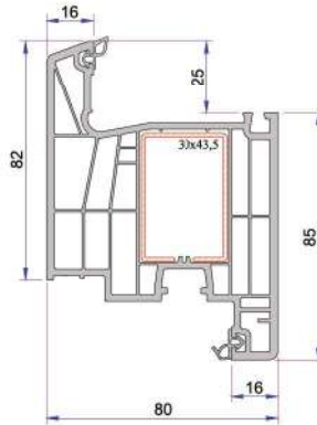
Kapı Kanat Profili (Kutu Destek Sacı) P.A.888.2113.600.2.BC.01
