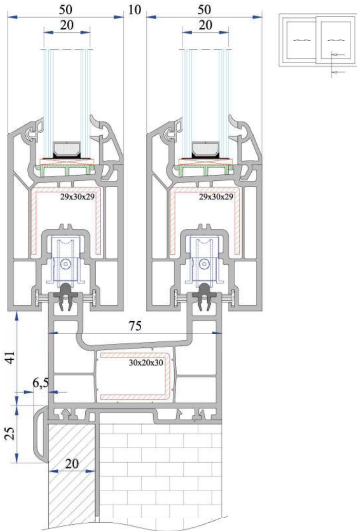
Kasa Altı Mantolama Profili Montajı
