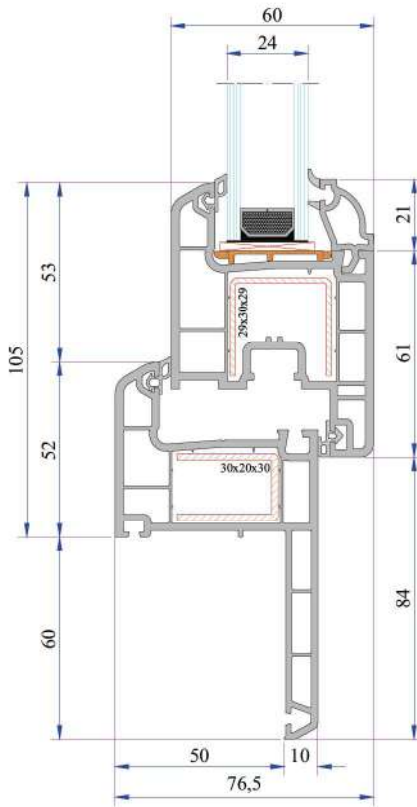
Pervazlı Kasa(60mm) - Kanat Profil Montajı
