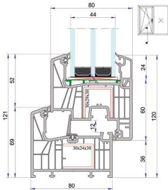
Kasa - Kanat Montajı
