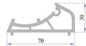
Açılı Dönüş Adaptörü Profili P.A.070.5104.600.0.00.19
