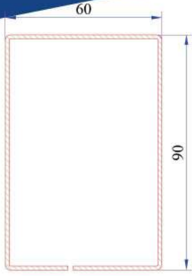
100mm Kutu Profili Destek Sacı 34022-12121
