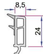
48mm Cam Çıtası P.A.888.4900.600.0.HC
