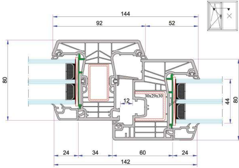
Orta Kayıt - Kanat Montajı
