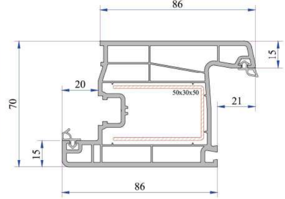
Kapı Kanat Profili P.A.750.2100.600.0.BC.01
