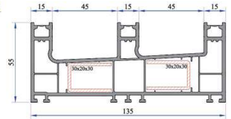
Kasa Profili (Üçlü Ray) P.A.232.1112.650.0.00.01
