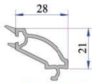
20 mm Dekoratif Çift Cam Çitası P.A.750.4102.600.0.HC
