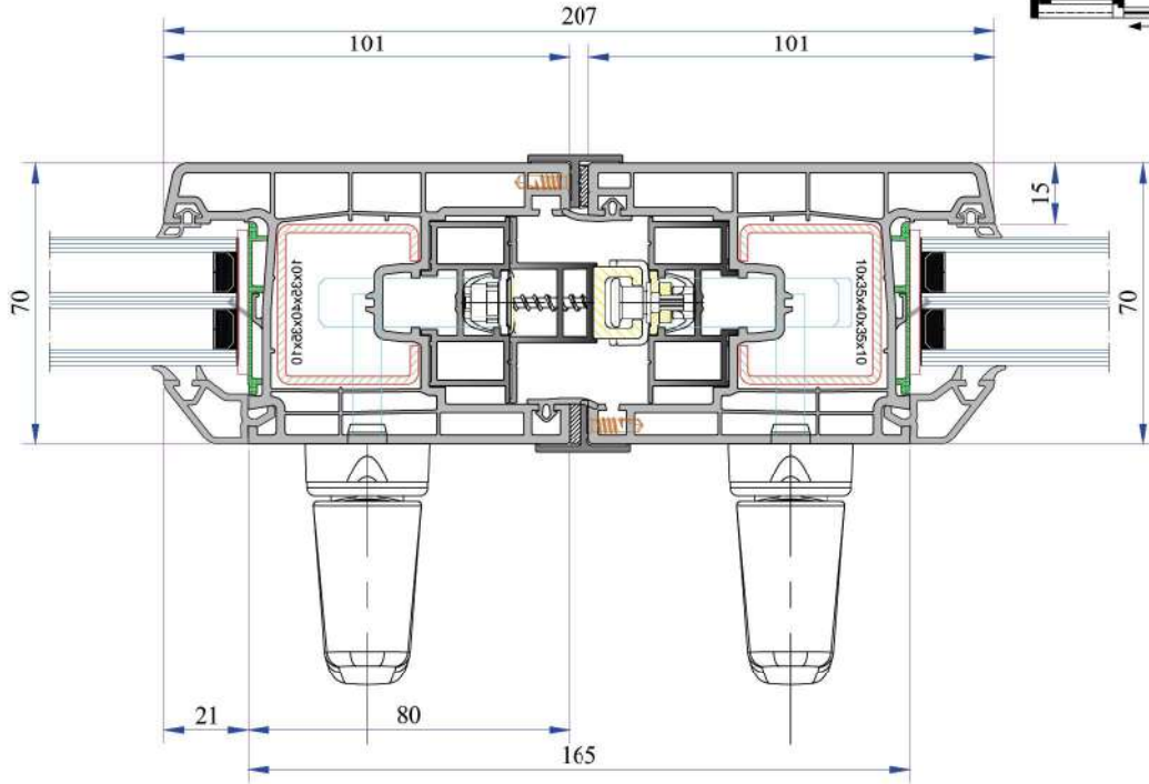
Çift Kanat Montajı
