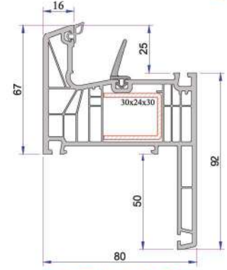
Pervazlı Kasa Profili P.A.888.1200.600.2.BC.01
