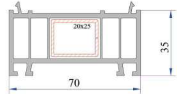
35mm Kasa Yükseltme Profili P.A.070.5300.600.0.00.19
