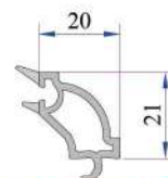
28 mm Dekoratif Contalı Çift Cam Çıtası P.A.101.4102.600.0.HC
