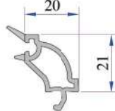
Contalı Çift Cam Çıtası 20 mm 101.4102
