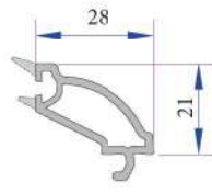
20mm Dekoratif Contalı Çift Cam Çıtası P.A.750.4102.600.0.HC
