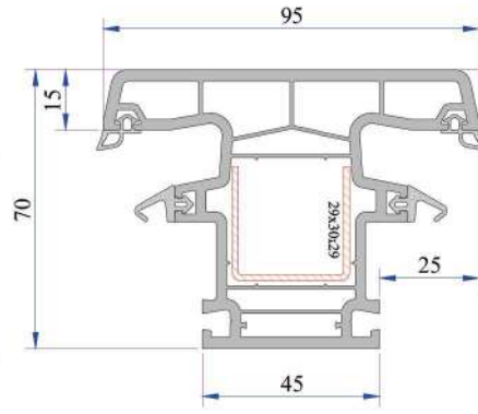
Orta Kayıt Profili P.A.777.3000.600.0.BC.01
