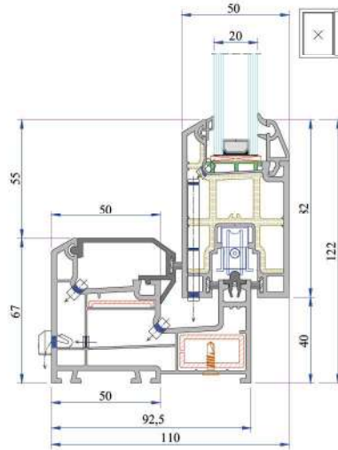
Tek Raylı Sürme Kasa - Kanat Montajı
