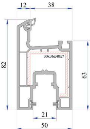
Sürme Kanat (Statik) P.A.232.2308.650.0.BC.01
