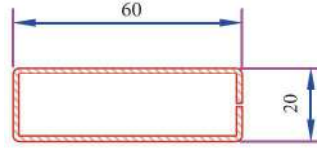
Kalın Bağ Profili Destek Sacı 34022 - 12106
