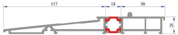
Hebeschiebe Alüminyum Isı Yalıtımlı Eşik 20mm (Yeni Yapılacak) AD16-079
