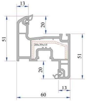
Dar Kanat Profil P.A.632.2003.600.0.BC.01
