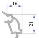
Dekoratif Çift Cam Çıtası 24 mm P.A.101.4202
