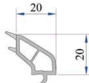
28 mm Contalı Çift Cam Çıtası P.A.101.4100.600.0.HC
