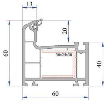
Kasa Profil P.A.632.1000.600.0.BC.01
