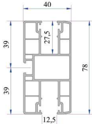
37'lik Lamel Orta Ray P.A.097.5603.600.0.00.19
