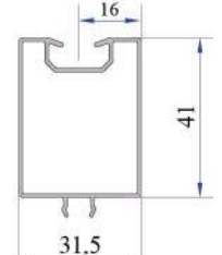
Panjur Yan Ray Yükseltme Ara Profili AD16-050
