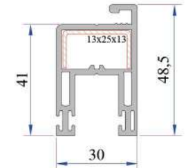
Sürme Sineklik Kanat P.A.242.2305.600.0.00.19
