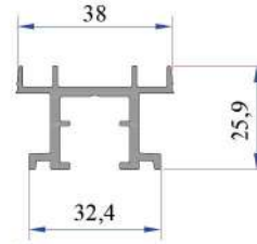
Kasa Üst Ray Alüminyum AD16-019
