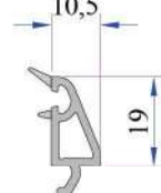
30mm Contalı Üçlü Cam Çıtası P.A.332.4100.600.0.HC
