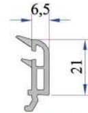
42 mm Üçlü Cam Çitası P.A.532.4500.600.0.HC
