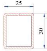
Orta Kayıt Profili Statik Destek Sacı 34022-12119
