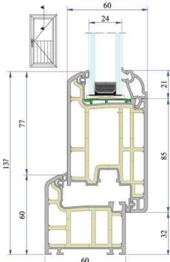
Kasa - Kapı Kanat Profil Montajı
