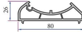
Açılı Köşe Dönüş Adaptörü P.A.080.5104.600.0.00.19
