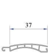
37'lik Lamel Yan Ray P.A.097.5602.600.0.00.19
