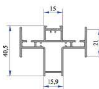
Alm. Kulaklı Çift kanat Ara Adaptörü (Yeni Yapılacak)
