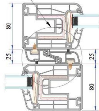
Hebeschiebe Kanat Ara Bindirme
