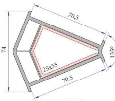
135° Köşe Profili P.A.070.5102.600.0.00.19
