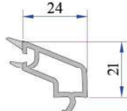
24 mm Contalı Çift Cam Çıtası P.A.750.4200.600.0.HC
