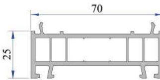
Kasa Yükseltme Profili 25 mm 070.5304
