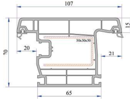
Dışa Açılım Kapı Kanat Profili P.A.750.2101.600.0.BC.01
