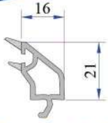
32 mm Contalı Üçlü Cam Çitası P.A.750.4500.600.0.HC
