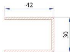
Eko Dışa Açılım Kapı Kanat Profili Destek Sacı 34022-12023
