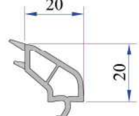
28 mm Contalı Çift Cam Çıtası 101.4100
