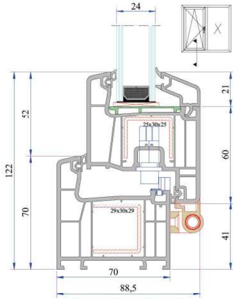
Kasa - Kanat Montajı
