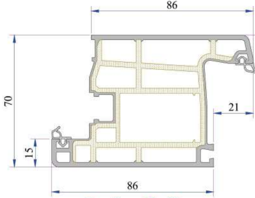
Kapı Kanat Profili P.A.750.2100.650.2.BC.35
