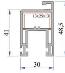
Sürme Sineklik Kanat Profili P.A.242.2305.600.0.00.03
