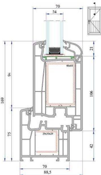
Kasa - Süper Kapı Kanat Montajı
