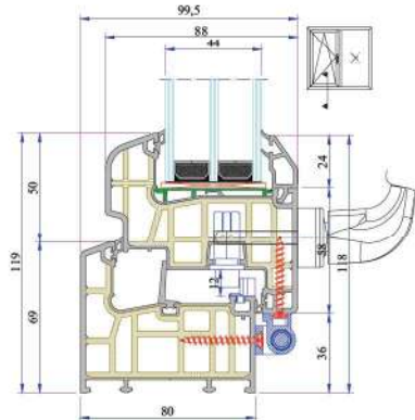
Kasa - Damlalıklı Kanat Montajı
