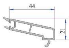
4-6 mm Contalı Tek Cam Çıtası P.A.750.4000.600.0.HC
