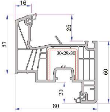
Kanat Profili P.A.888.2000.600.2.BC.01
