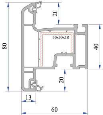
22 Aks Dışa Açılım Kanat Profil P.A.632.2014.600.0.BC.01
