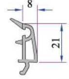
40 mm Üçlü Cam Çitası 101.4500.600.0.HC
