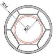
Açılı Dönüş Borusu Ø70mm P.A.070.5106.600
