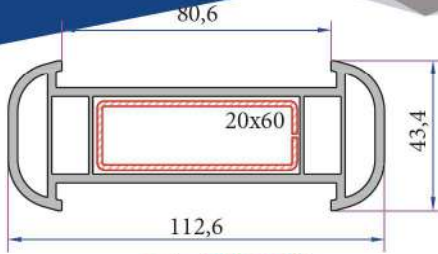
Kalin Baş Profili P.A.080.5000.600.0.00.19
