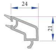
24mm Contalı Çift Cam Çıtası P.A.750.4200.600.0.HC
