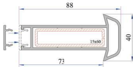
Universal Kalın Bağ Profili Kapağı 058.5000
