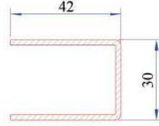
Eko Kapı Kanat - Dışa Açılım Eko Kapı Kanat Profili Destek Sacı 34022-12023
