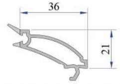
4-6mm Contalı Tek Cam Çıtası P.A.101.4002.600.0.HC
