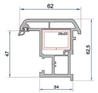
Hareketli Orta Kayıt Profili P.A.632.3100.0
