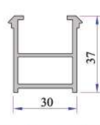
Kasa Montaj Profili P.A.060.5301.600.0.00.19
