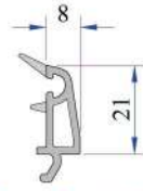
40 mm Contalı Üçlü Cam Çitası P.A.101.4500.600.0.HC
