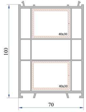
100mm Kasa Yükseltme Profili P.A.070.5302.600.0.00.19
