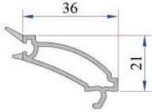
Contalı Tek Cam Çıtası 4-6 mm 101.4002
