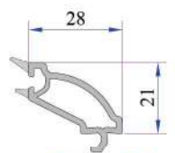
20 mm Dekoratif Contalı Çift Cam Çıtası P.A.750.4102.600.0.HC
