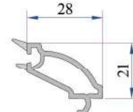
20 mm Dekoratif Contalı Çift Cam Çıtası P.A.750.4102.600.0.HC
