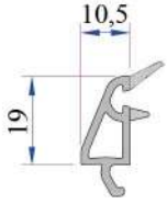
20mm Çift Cam Çıtası P.A.332.4100.600.0.0.HC
