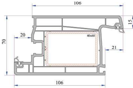
Süper Kapı Kanat Profili P.A.750.2103.600.0.BC.01
