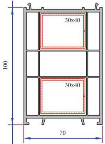
100mm Kasa Yükseltme Profili P.A.070.5302.600.0.00.19
