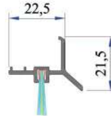
Açılı Köşe Dönüş Adaptörü P.A.080.5104.600.0.00.19
