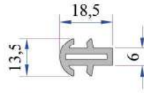
İnce Bağ Profili 099.5003
