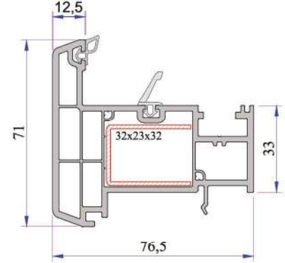
Hareketli Orta Kayıt Profili P.A.888.3100.600.2.BC.01
