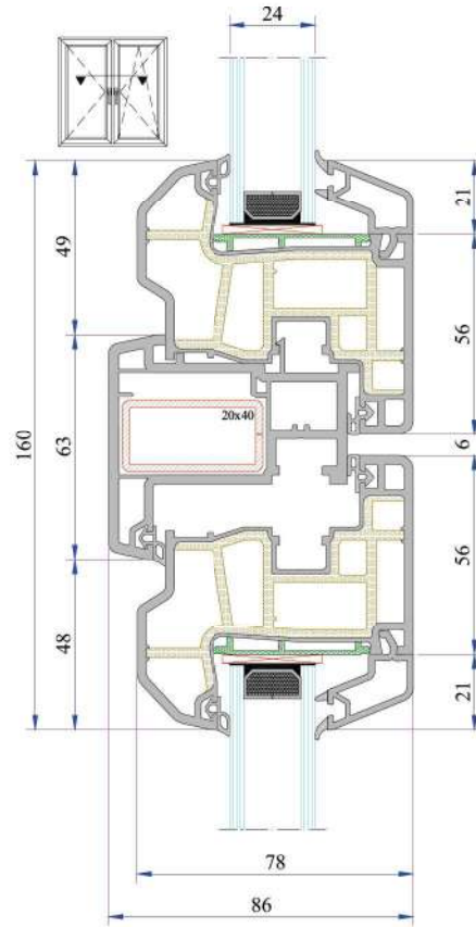
Damlalıklı Kanat - Hareketli Orta Kayıt Montajı
