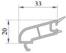
24mm Çift Cam Çitası P.A.800.4200.600.0.HC
