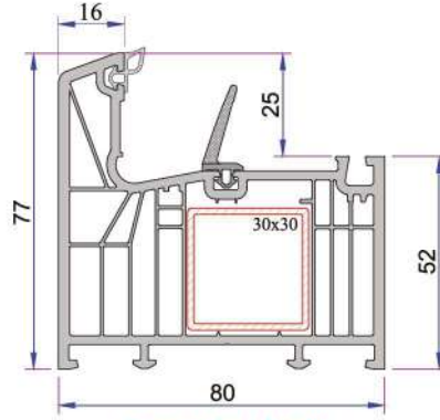
Süper Kasa Profili P.A.888.1001.600.2.BC.01
