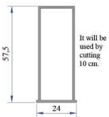
Alüminyum Kanat Yataklama Profili AD16-083
