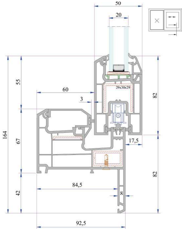
Tek Raylı Pervazlı Sürme Kasa - Sürme Kanat Montajı
