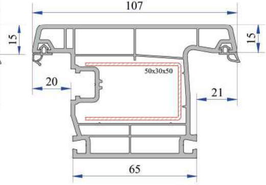
Dışa Açılım Kapı Kanat Profili P.A.750.2101.650.0.BC.35
