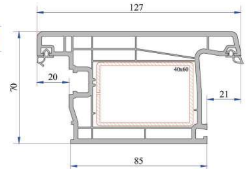
Dışa Açılım Süper Kapı Kanat Profili P.A.752.2104.600.0.BC.03
