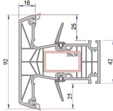
Orta Kayıt Profili P.A.888.3000.600.2.BC.01
