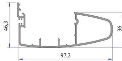
Kanat Kapama Griyaj Profili AD16-028
