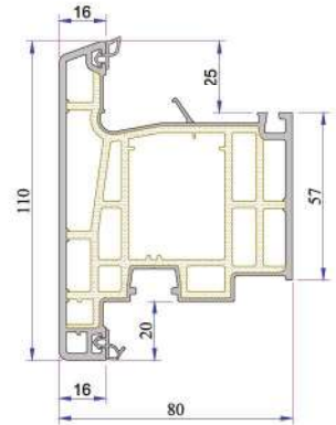
Dışa Açılım Kapı Kanat Profili Penwood P.A.888.2101.600.2.BC.01
