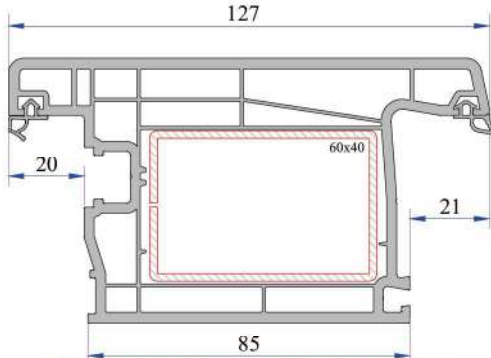
Dışa Açılım Süper Kapı Kanat Profili P.A.750.2104.650.0.BC.35
