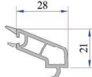
20 mm Contalı Çift Cam Çıtası P.A.750.4100.600.0.HC
