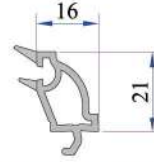
32 mm Dekoratif Üçlü Cam Çitası P.A.750.4201.600.0.HC
