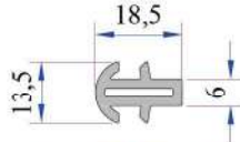
Kısa Bağ Profili P.A.099.5003
