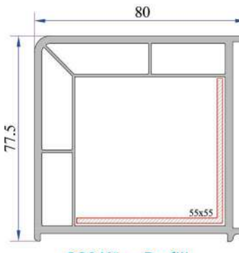
90° Köşe Profili P.A.070.5100.600.0.00.19
