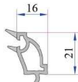
32 mm Dekoratif Contalı Üçlü Cam Çıtası 101.4202
