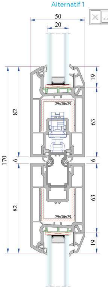
Alm. Çift Ray Adaptörü (Dörtlü Kanat Ara Profili)
