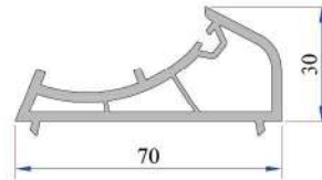
Açılı Dönüş Adaptör Profili P.A.070.5104.600.0.00.19
