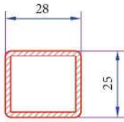
Hareketli Orta Kayıt Destek Sacı 34022-12117
