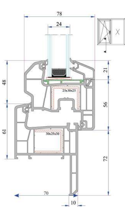
Pervazlı Kasa - Kanar Montajı
