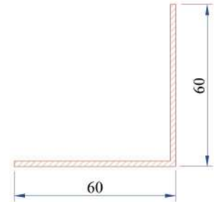
90° Köşe Dönüş Profili Destek Sacı 34022-12306
