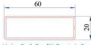
Kalın Bağ Profili Destek Sacı 34022-12106
