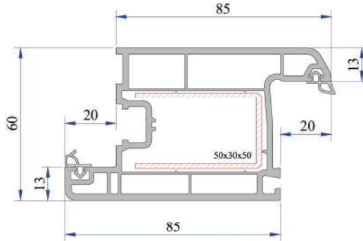
Kapı Kanat Profil P.A.632.2100.650.0.BC.01
