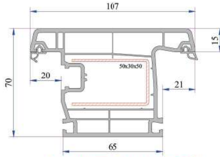
Dışa Açılım Kapı Kanat Profili P.A.750.2101.650.0.BC.01
