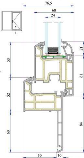
Pervazlı Kasa - Kanat Profil Montajı
