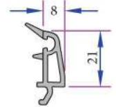
40mm Contalı Üçlü Cam Çıtası P.A.101.4500.600.0.HC
