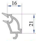
32 mm Dekoratif Contalı Üçlü Cam Çitası P.A.101.4202.600.0.HC
