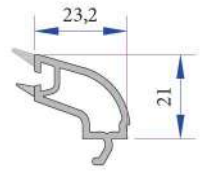
24mm Dekoratif Contalı Çift Cam Çıtası P.A.750.4204.600.0.HC
