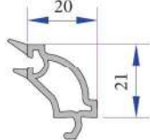
28mm Dekoratif Contalı Çift Cam Çıtası P.A.101.4102.600.0.HC
