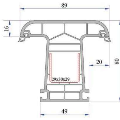
Orta Kayıt Profili P.A.860.3000.600.0.BC.01
