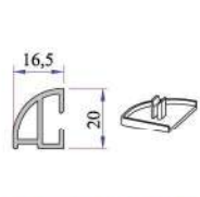
Damlalıklı Profil P.A.900.5106.600.0.00.19
