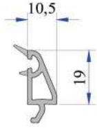
Dekoratif Üçlü Cam Çitası 30 mm P.A.332.4100
