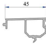
Tek Ray Kanal Kapama Profili P.A.232.5710.600.0.0.HC
