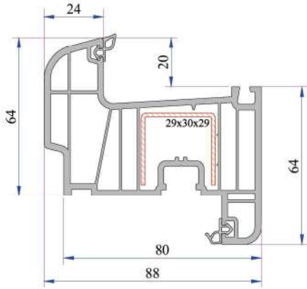
Damalıklı Kanat Profili P.A.860.2200.600.0.BC.01
