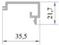
Kanat İç Kapatma Profili P.A.098.5905
