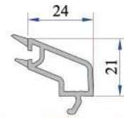
24 mm Çift Cam Çitası P.A.750.4200.600.0.HC
