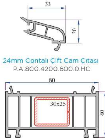
Kasa Yükseltme Profili P.A.080.5300.600.0.00.19
