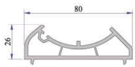
Açılı Dönüş Adaptör Profili P.A.080.5104.600.0.00.19
