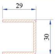
Kasa - Kanat - Orta Kayıt Profili Destek Sacı 34022-12002
