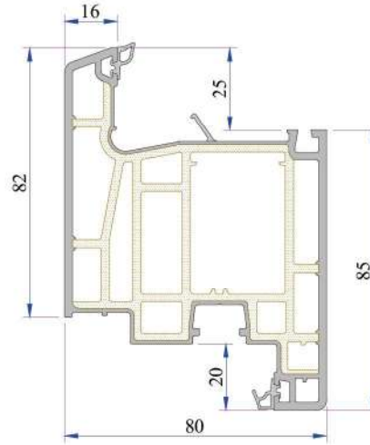
Kapı Kanat Profili P.A.883.2100.2
