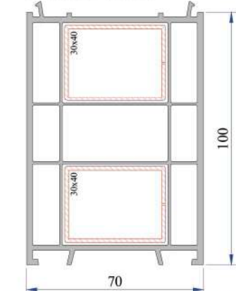
100mm Kasa Yükseltme Profili P.A.070.5302.600
