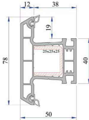
332 Orta Kayıt Profili P.A.332.3000
