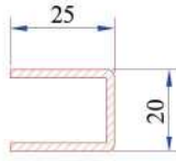
Pervazlı Kasa Profili Destek Sacı 34022-12021
