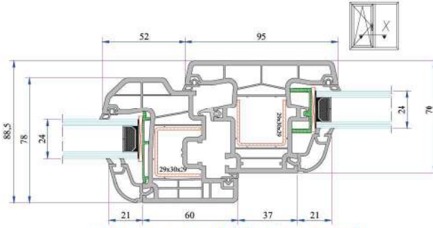
Orta Kayıt - Damlalıklı Kanat Montajı
