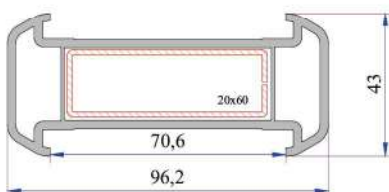
Kalın Bağ Profili P.A.070.5000.600.0.00.19
