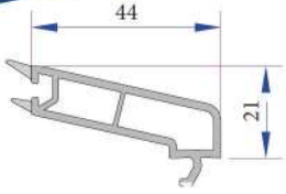
4-6mm Contalı Tek Cam Çıtası P.A.750.4000.600.0.HC
