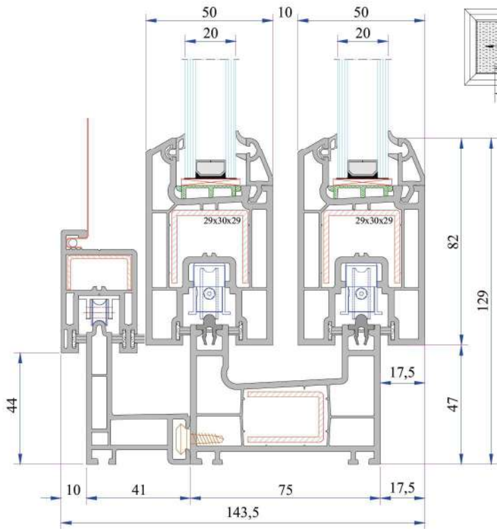
Çift Ray Sürme Kasa - Sürme Kanat - Sineklik Ray Profili Montajı Detayı
