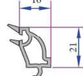
32mm Dekoratif Contalı Üçlü Cam Çıtası P.A.101.4202.600.0.HC
