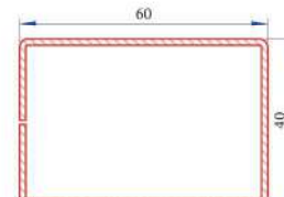
Super Statik Orta Kayıt Destek Sacı 34022-12110
