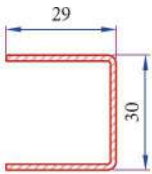
Kasa, Kanat, Orta Kayıt Destek Sacı 34022-12002
