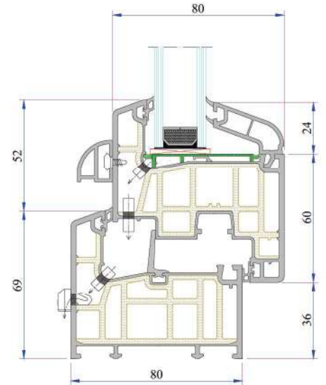
Damlalıklı Profili Montajı
