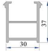
Kasa Montaj Profili P.A.060.5301
