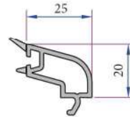
Contalı Üçlü Cam Çıtası 32mm P.A.800.4500.600.0.HC
