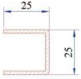
Kasa - Orta Kayıt Profili Destek Sacı 34022-12003
