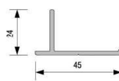
Geniş T Profili P.A.099.5508
