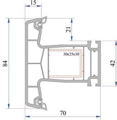
Kapı İçi Orta Kayıt Profili P.A.750.3000.600.0.BC.01
