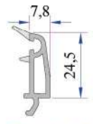
40 mm Contalı Üçlü Cam Çitası P.A.433.4500.600.0.HC
