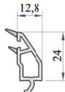
44mm Cam Çıtası P.A.888.4800.600.0.HC
