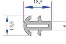
Kısa Bağ Profili P.A.099.5003.600
