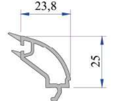
32-34mm Cam Çıtası P.A.777.4204.600.0.HC
