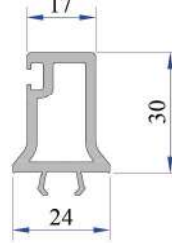
Hebeschiebe Kasa Orta Adaptörü P.A.900.6503.600.0.HC
