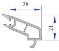
20mm Contalı Çift Cam Çıtası P.A.750.4100.600.0.HC
