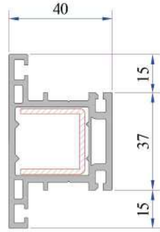
Kanat Profili P.A.098.5900.600.0.00.19
