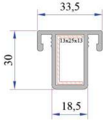
Sürme Sineklik Orta Kayıt P.A.242.3200.600.0.00.19
