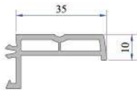
Kasa Altı Klips Pervaz (35mm) P.A.099.5523
