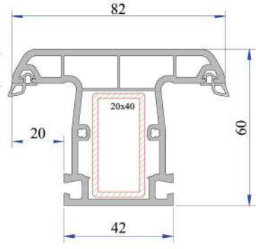
Statik Orta Kayıt Profil 900.3003
