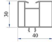
Panjur Yan Ray Yükseltme Ara Profili 21108-01000
