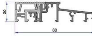
Yalıtımlı Eşik Profili AD16-089
