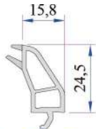
42mm Cam Çıtası P.A.777.4302.600.0.HC
