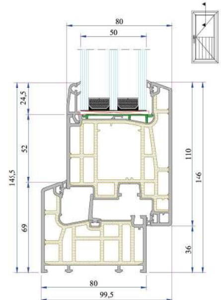
Kasa - Dışa Açılım Kapı Kanat Montajı
