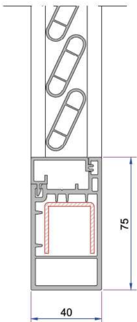
KepenK Kanat Lamel Uygulaması
