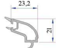
24 mm Dekoratif Contalı Çift Cam Çıtası P.A.750.4204.600.0.HC
