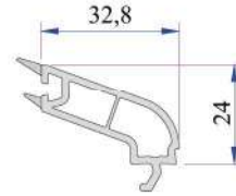
24mm Cam Çıtası P.A.883.4204.600.0.HC
