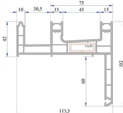
Sürme Pervazlı Sineklik Kasa (60mm Pervaz) P.A.232.1115.650.0.BC.01
