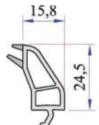
42mm Cam Çıtası P.A.777.4302.600.0.HC
