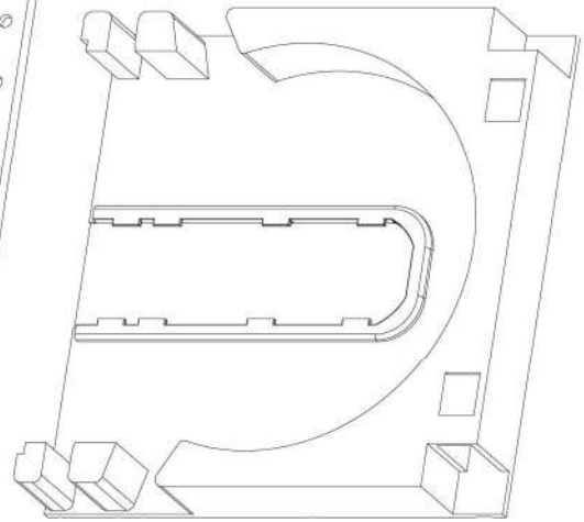
190x190mm Panjur Orta Kapak 34019-11240
