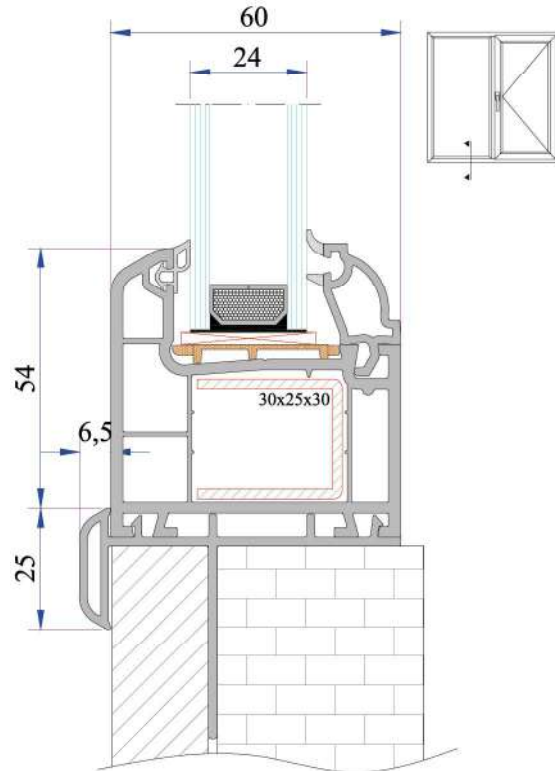
Kasa Altı Mantolama Profili Montajı
