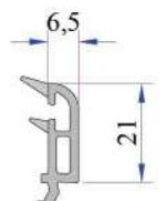
42 mm Contalı Üçlü Cam Çıtası 532.4500
