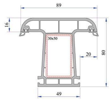
Statik Orta Kayıt Profili P.A.800.3009.600.0.BC.01
