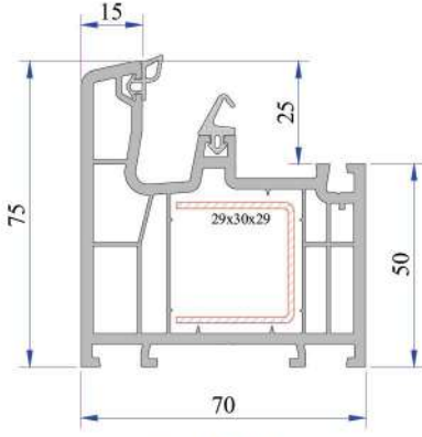
Kasa Profili P.A.777.1000.600.0.BC.01
