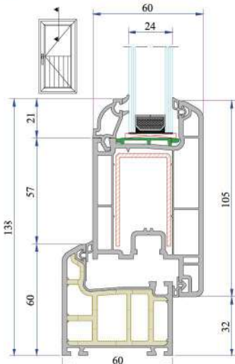
Kasa - Dışa Açılım Kapı Kanat Profil Montajı
