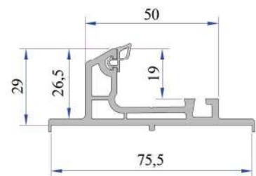
Çift Ray Adaptör Profili P.A.232.5800.650.0.BC.19
