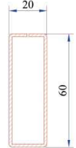
Kalın Baş Profili Destek Sacı 34022-12106
