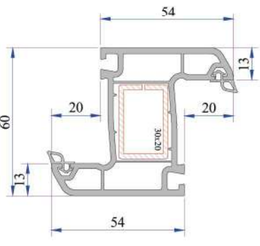
Dışa Açılım Orta Kayıt Profil P.A.632.3005.600.0.BC.01
