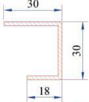
Dışa Açılım Kanat Profili Destek Sacı 34022-12022
