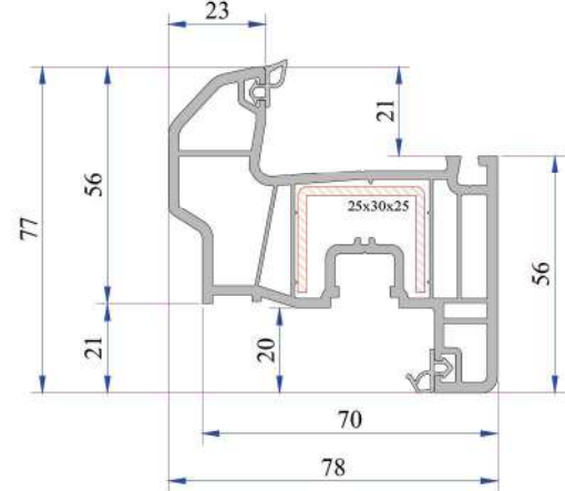
Damlalıklı Kanat Profili P.A.750.2200.600.0.BC.01
