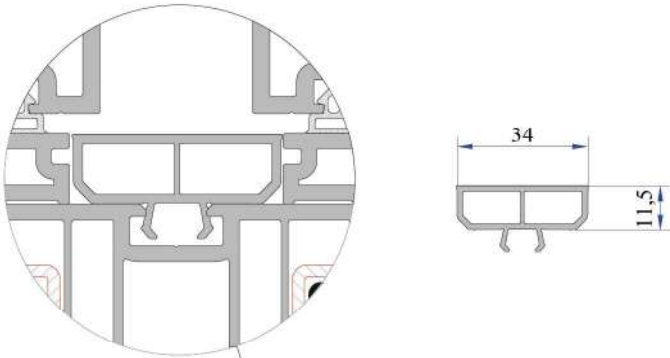
Hebeschiebe Kasa Orta Adaptörü Montajı
