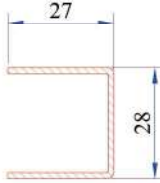
Dışa Açılım Kanat Profili Destek Sacı (9 Aks) 34022-12020
