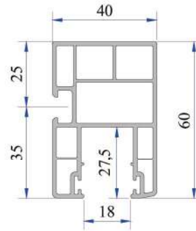
55'lik Lamel Yan Ray P.A.097.5613.600.0.00.19
