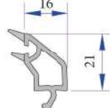
32mm Contalı Üçlü Cam Çıtası P.A.750.4500.600.0.HC
