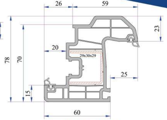
Damlalıklı Kanat Profili P.A.777.2000.600.0.BC.01
