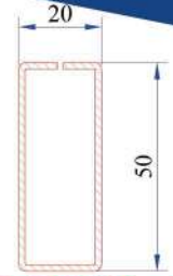
Kalın Bağ Profili Destek Sacı 34022-12105
