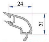
24 mm Dekoratif Çift Cam Çitası P.A.750.4204.600.0.HC
