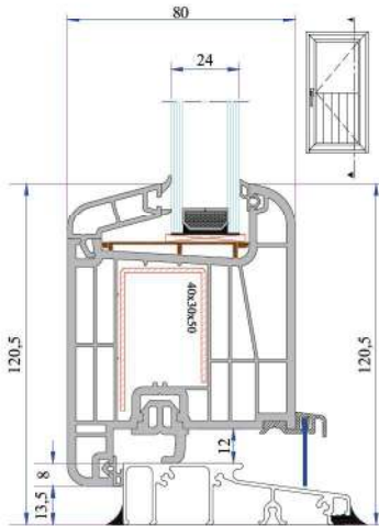
Alüminyum Eşikli Kapı Kanat Montajı
