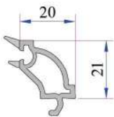
28 mm Dekoratif Contalı Çift Cam Çıtası 101.4102
