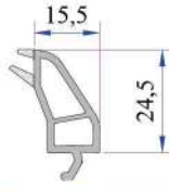
32 mm Contalı Üçlü Cam Çitası P.A.433.4200.600.0.HC
