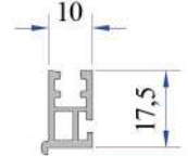
PVC Tampon Çıtası P.A.097.5605.600
