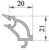
28 mm Dekoratif Çift Cam Çitası P.A.101.4102.600.0.HC
