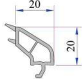
Contalı Çift Cam Çıtası 20 mm 101.4100
