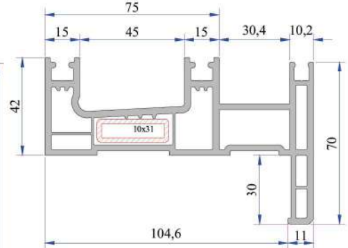
Pervazlı Sineklikli Kasa P.A.242.1104.650.0.00.01
