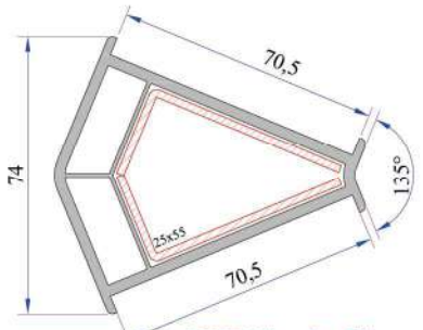
135° Köşe Profili P.A.070.5102.600.0.00.19
