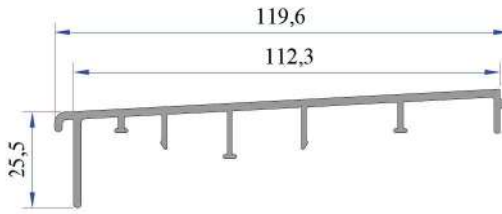
Alüminyum Eşik Kapama AD16-024
