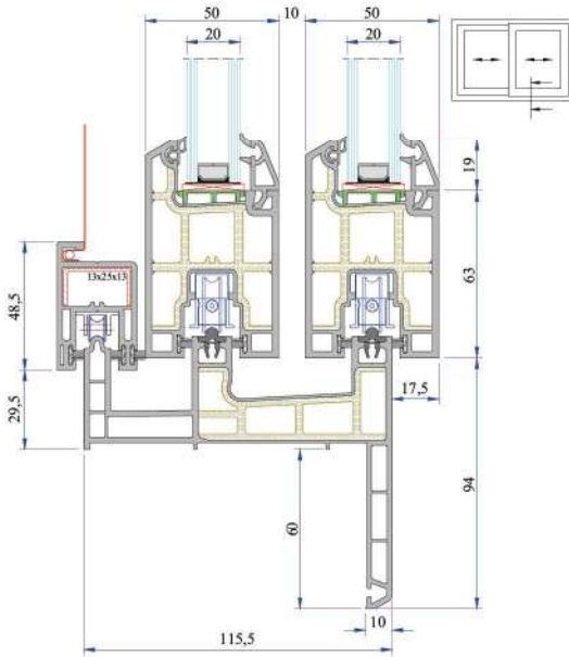
60mm Sürme Pervazlı Sineklik Kasa - Kanat Montajı
