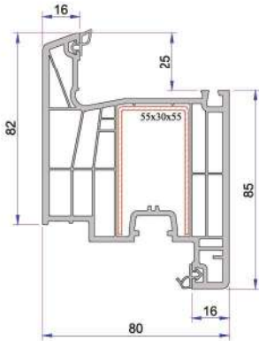
Kapı Kanat Profili P.A.888.2100.600.2.BC.01
