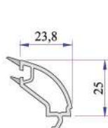
32-34mm Cam Çıtası P.A.777.4204.600.0.HC
