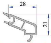
20 mm Çift Cam Çitası P.A.750.4100.600.0.HC
