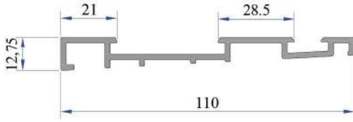
Alüminyum Eşik İkinci Kanat Ray AD16-025
