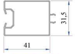
Panjur Yan Ray Yükseltme Ara Profili AD16-050
