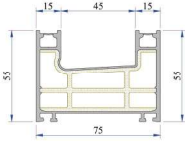
Çift Raylı Kasa Profili P.A.232.1106.2
