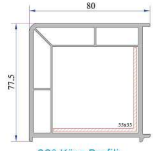
90° Köşe Profili P.A.070.5100.600.0.00.19
