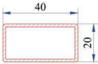
Kasa Profili Destek Sacı 34022-15114
