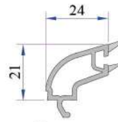
32mm Üçlü Cam Çitası P.A.750.4204.600.0.HC
