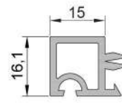
Kasa Altı Pervaz Profili 15mm P.A.099.5525
