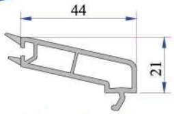
4-6 mm Cam Çitası P.A.750.4000.600.0.HC
