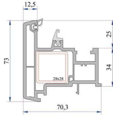
Hareketli Orta Kayıt Profili P.A.777.3100.600.0.BC.19
