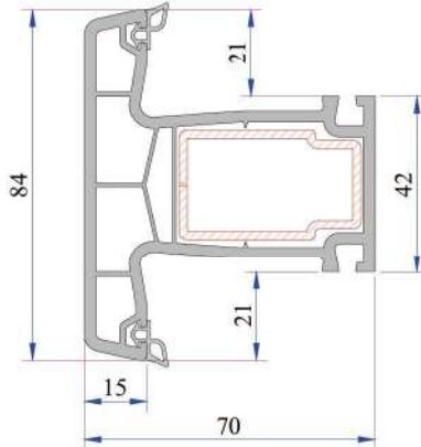
Statik Orta Kayıt Profili P.A.750.3007.600.0.BC.01
