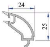
24 mm Dekoratif Contalı Çift Cam Çıtası P.A.777.4204.600.0.HC
