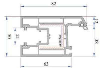
Sürme Kanat P.A.232.2300.650.0.BC.01
