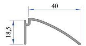
20mm Eşik İç Profili (Yeni Yapılacak) AD16-080
