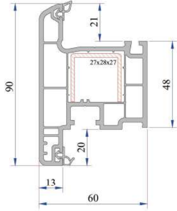
9 Aks Dışa Açılım Kanat Profil 430.2001
