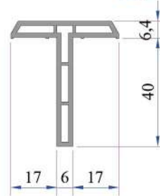
KepenK T Profili P.A.098.5902
