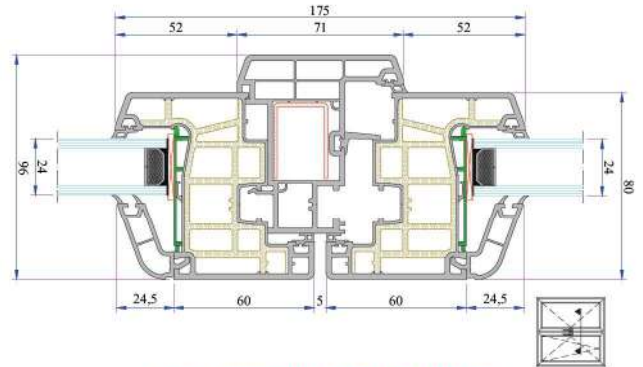
Kanat-Hareketli Orta kayıt Montajı
