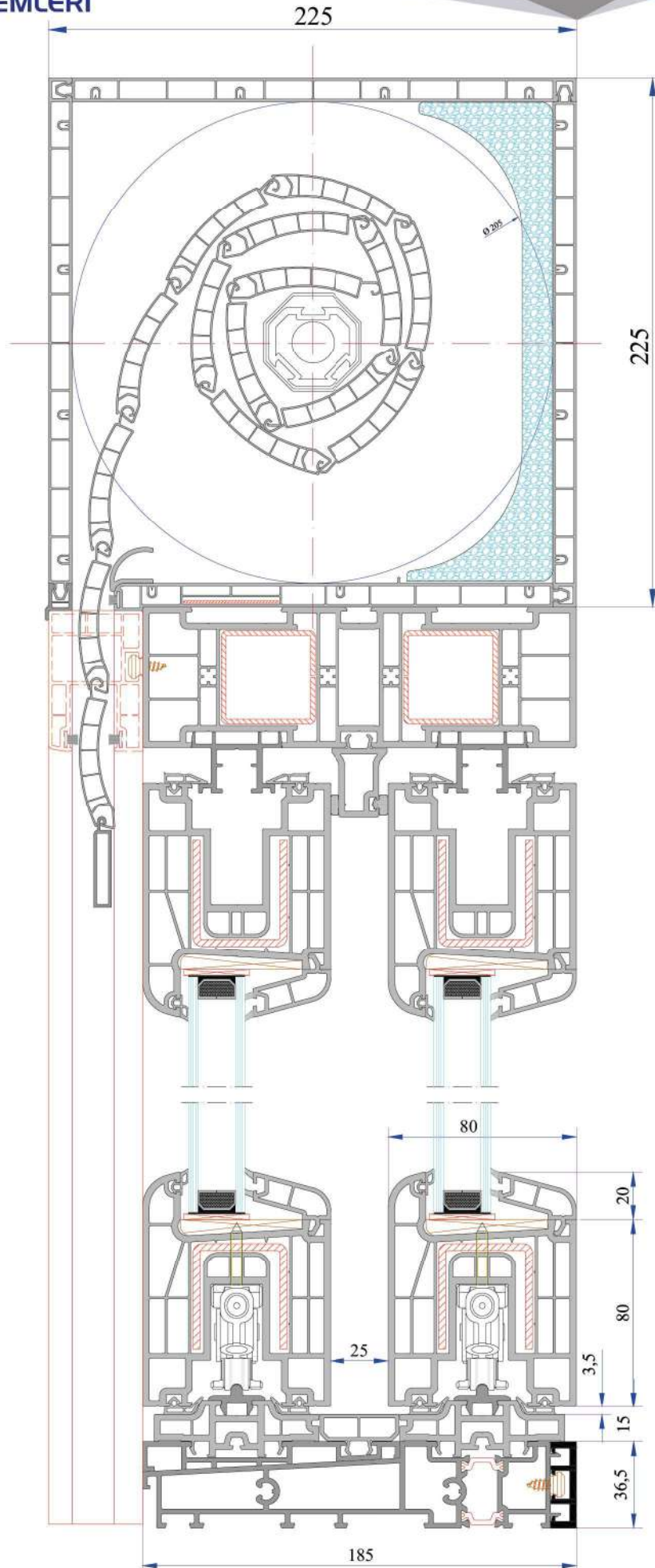
Hebeschiebe Sürme Sisteminde 225x225mm Panjur Kutu Uygulaması (55-37-39-40mm'lik Lamel uygulanabilmektedir.)
