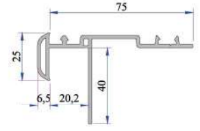
Kasa Altı Mantolama Profili P.A.099.5548.600.0.0.HC
