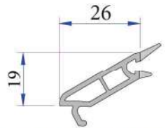
Tek Cam Çıtası (4mm) 332.4000
