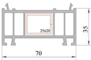
35mm Kasa Yükseltme Profili P.A.070.5300.600.0.00.19
