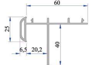
Kasa Altı Mantolama Profili 099.5545
