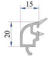
42mm Üçlü Cam Çitası P.A.800.4600.600.0.HC
