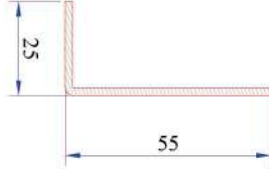
135° Köşe Profili Destek Sacı 34022-12303
