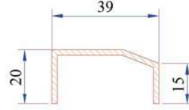
Dar Kanat Profili Destek Sacı 34022-12031
