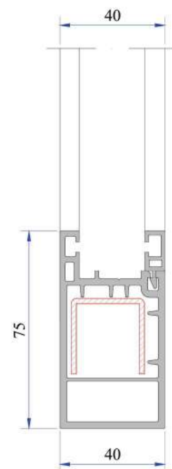
KepenK Kanat Lamel Uygulaması
