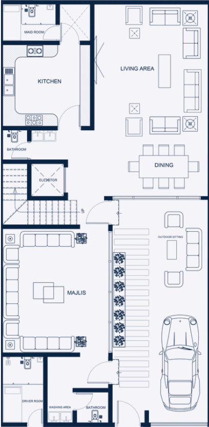
الأرضي Ground Floor
