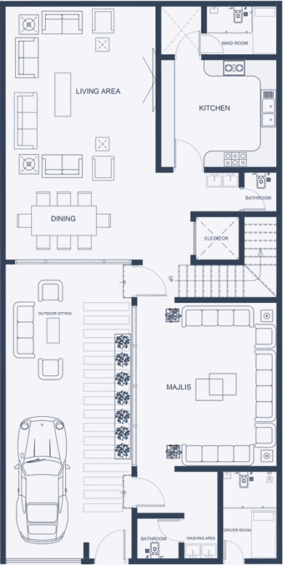
الأرضي Ground Floor
