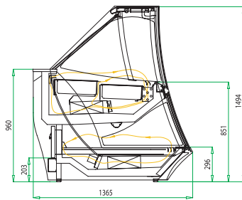
SEZIONE SOFIA ALTA GELATERIA SOFIA ICE CREAM HIGH GLASSES SECTION
