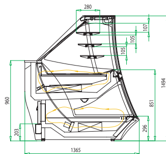
SEZIONE SOFIA ALTA PASTICCERIA SOFIA PASTRY HIGH GLASSES SECTION
