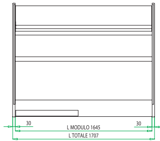
PIANTA MODULO 170 MODULE 170 LAYOUT
