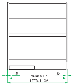
PIANTA MODULO 120 MODULE 120 LAYOUT
