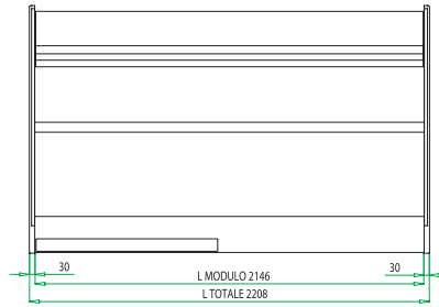
PIANTA MODULO 220 MODULE 220 LAYOUT
