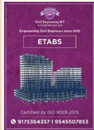
ETABS
