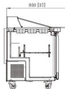
TSSU-72MT
