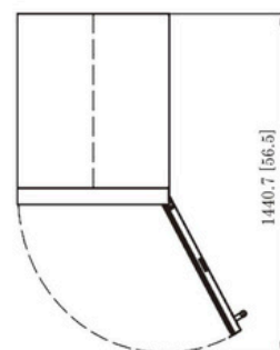
Door open size
