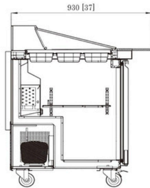
TSSU-29MT
