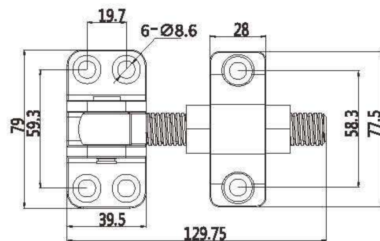
合页型 CH402-3
