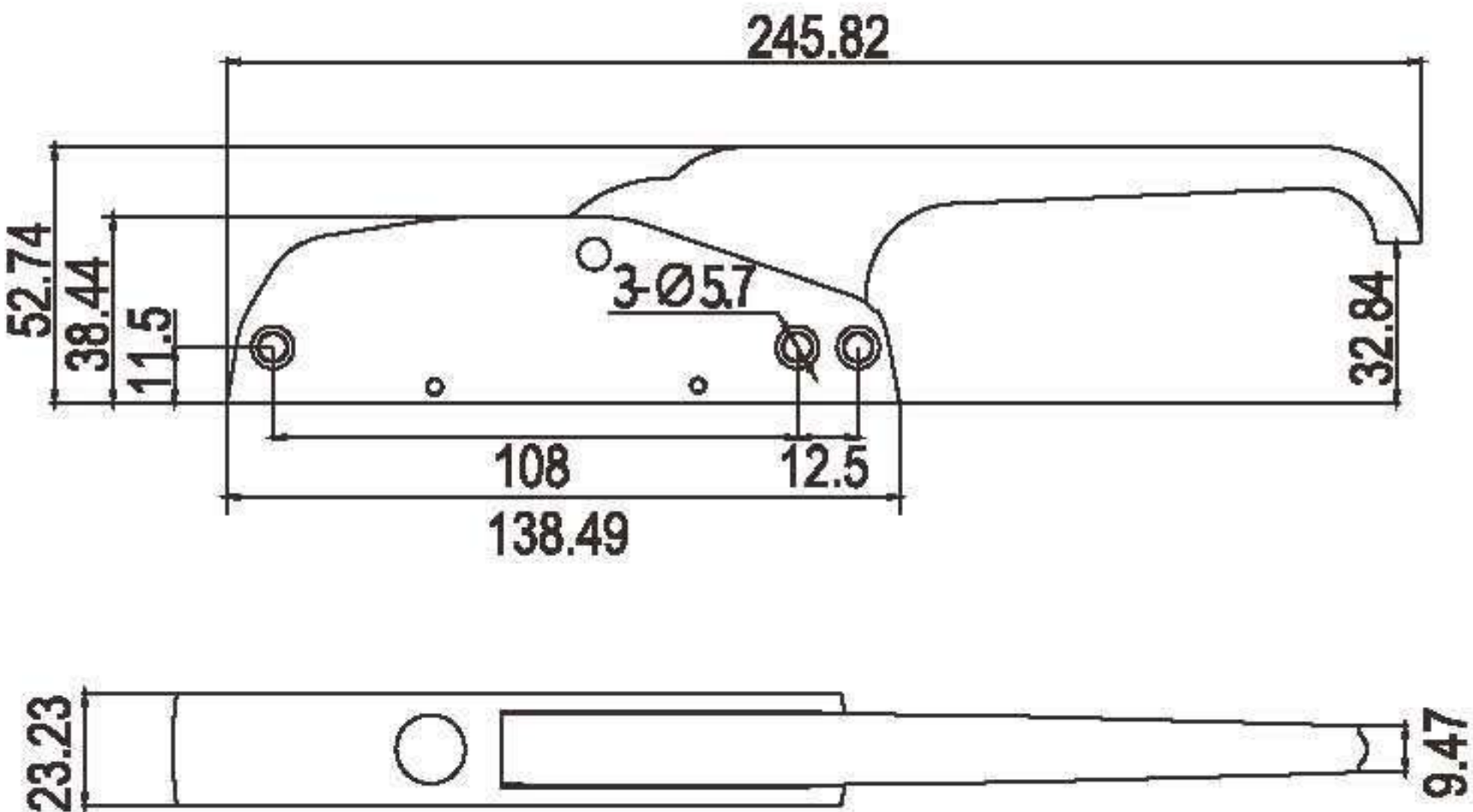
把手尺寸
