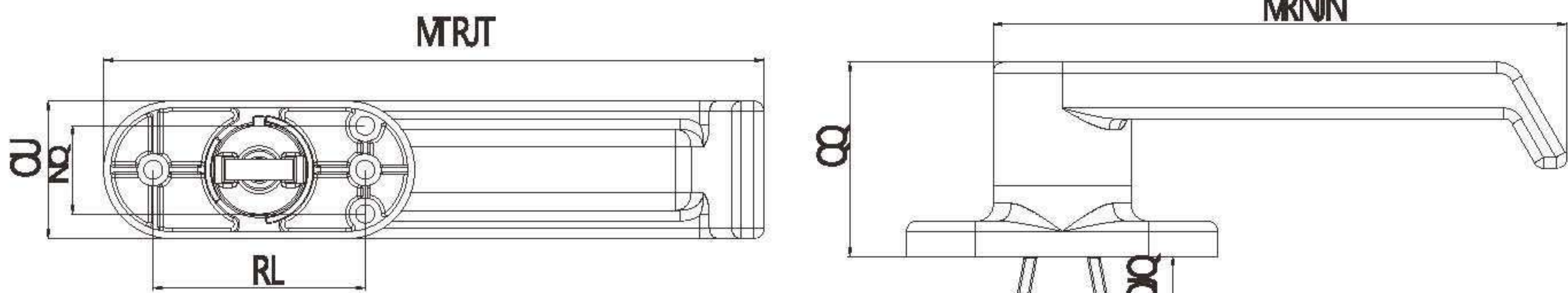
把手尺寸
