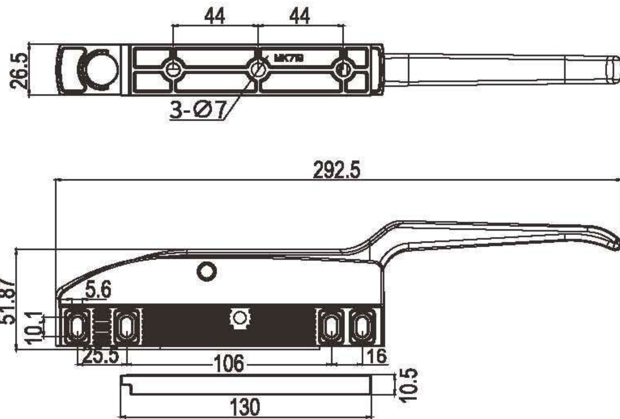
CH719-2 保温车把手 (无锁芯)
