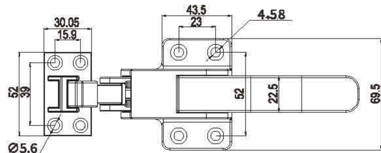
CH703-3 锌合金
