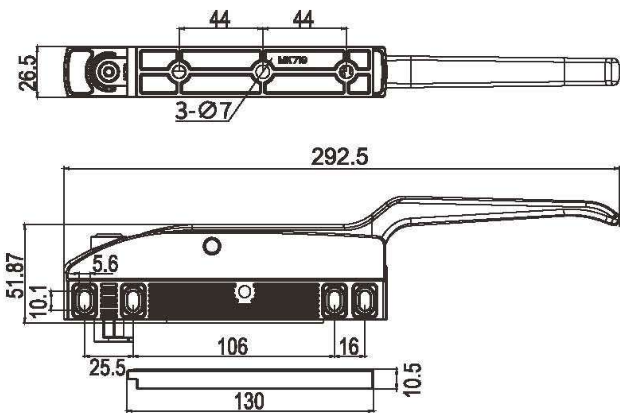
CH719-1 保温车把手 (有锁芯)
