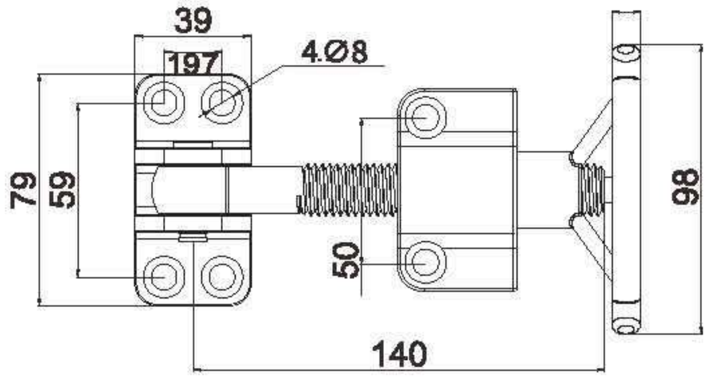
固定型 CH401-2
