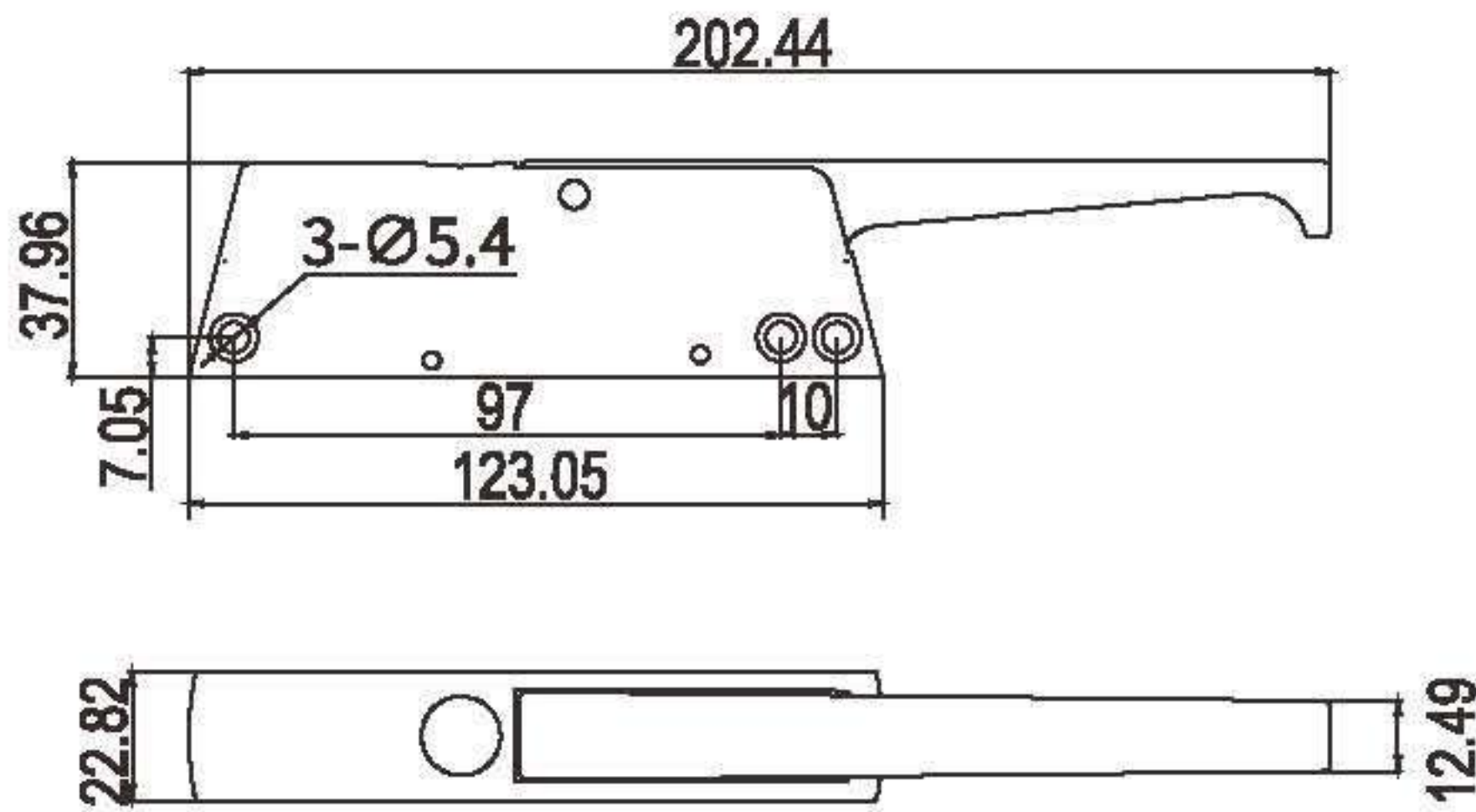
把手尺寸
