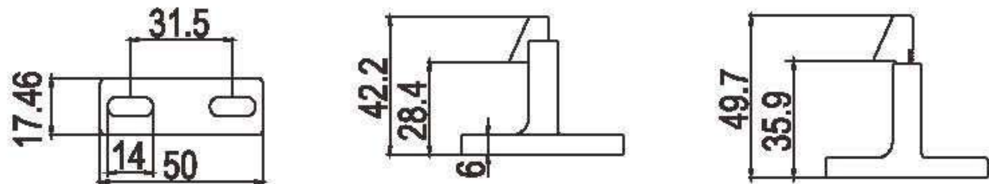
扣子尺寸
