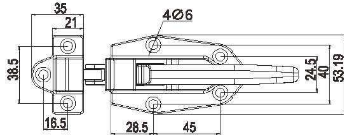
CH701-3 锌合金
