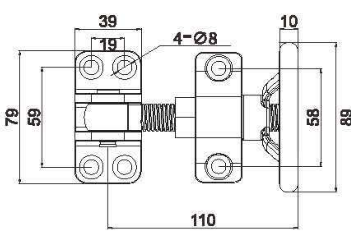
固定型 CH402-2
