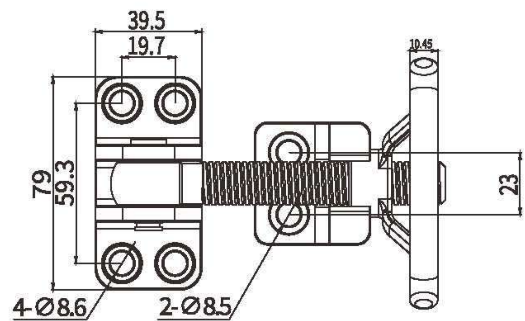
M16防滑手轮活动款
