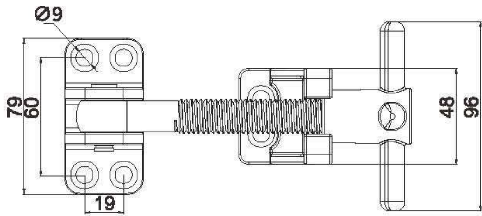
活动手轮 SY1-0405-1
