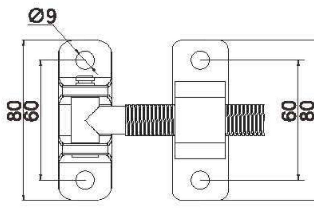
轻型合页 CH403-4
