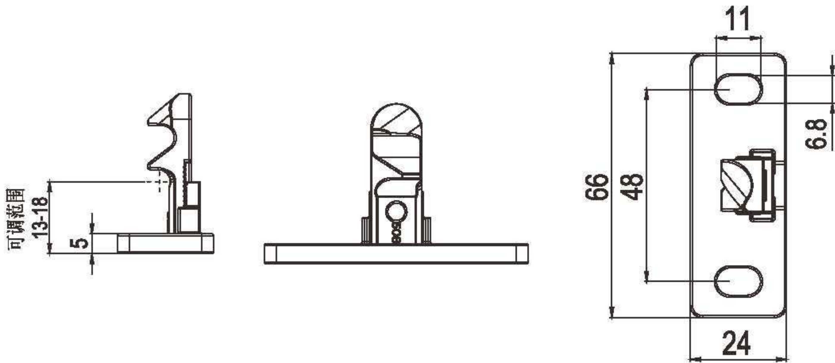
CH508 双级门扣
