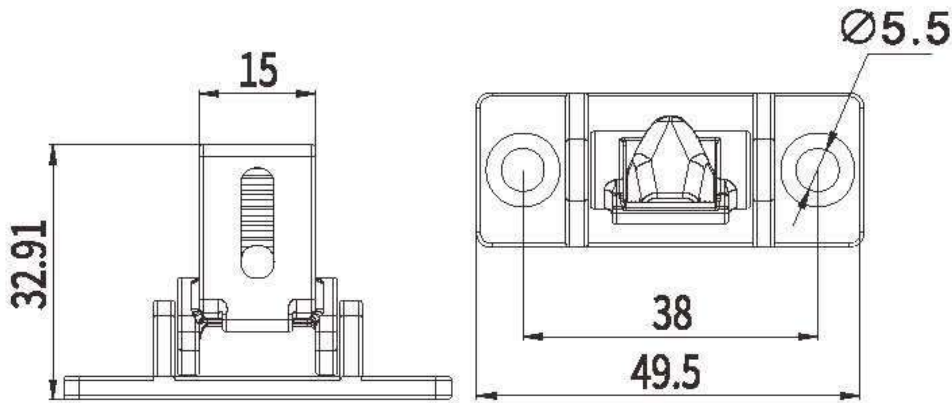
扣子
