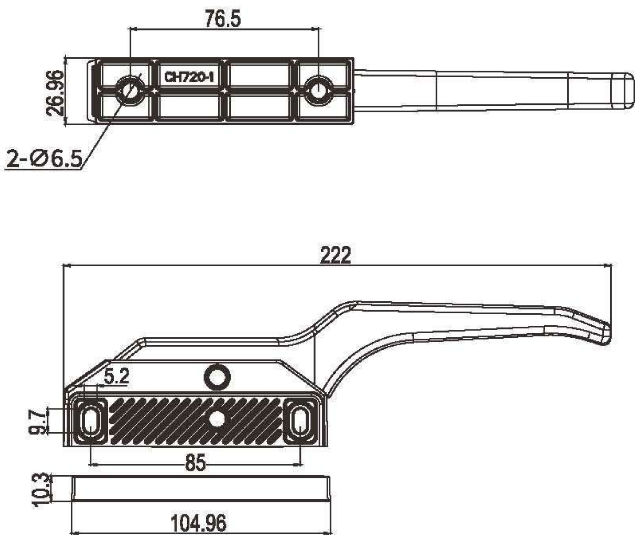
CH720 保温车把手
