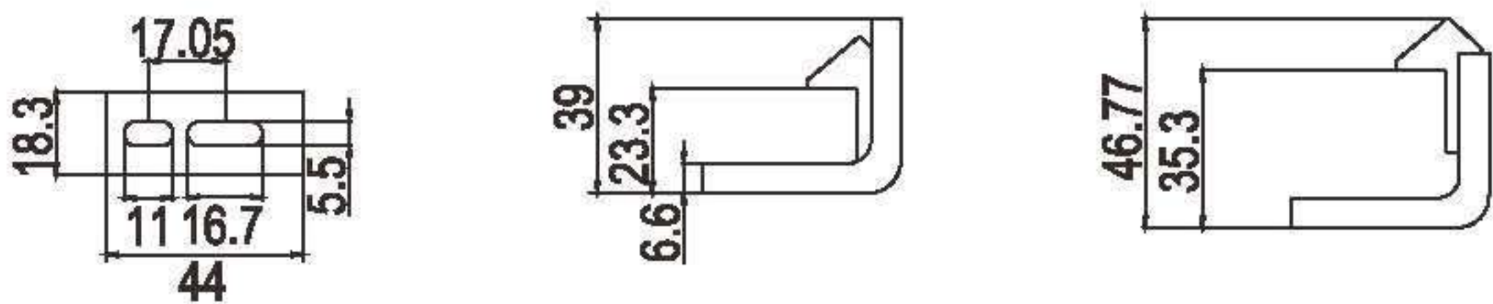
扣子尺寸
