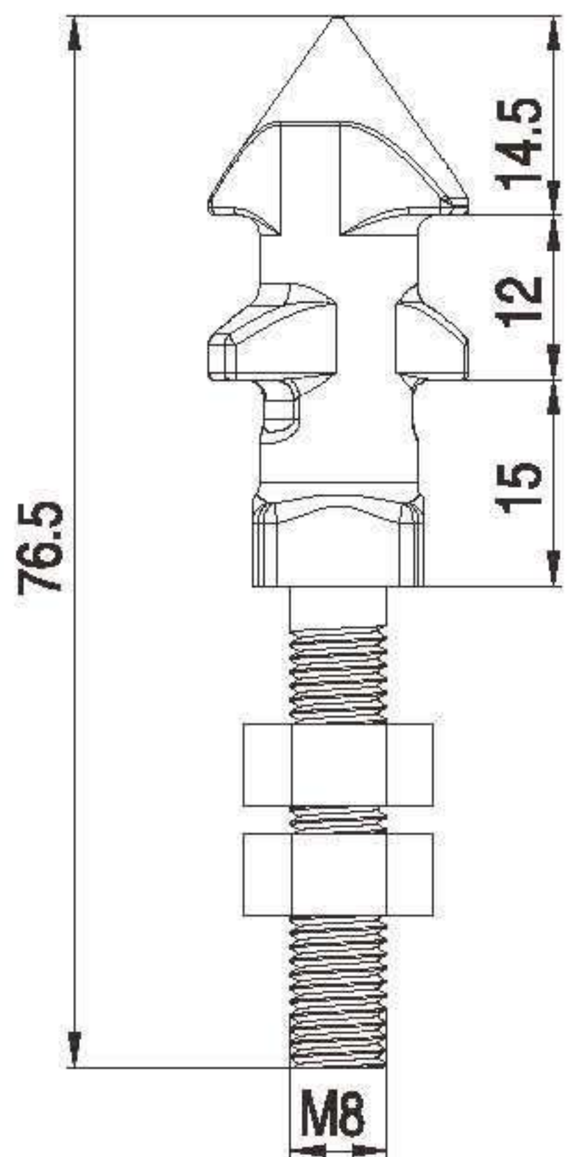
调节扣尺寸
