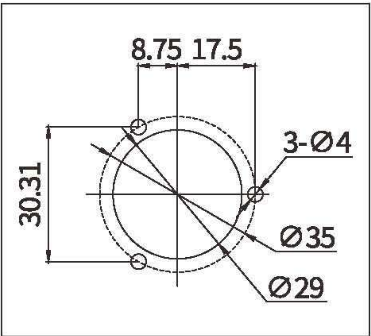
门板开孔尺寸
