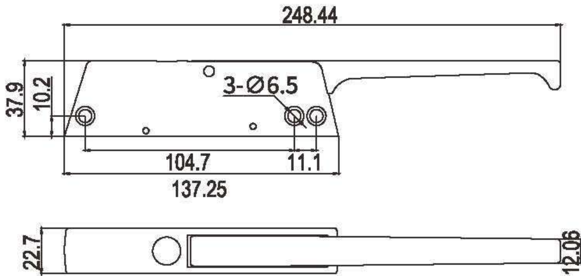
把手尺寸
