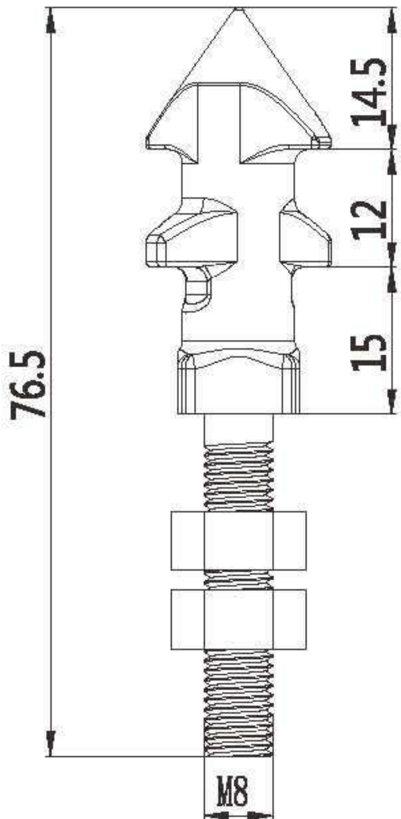
调节扣尺寸
