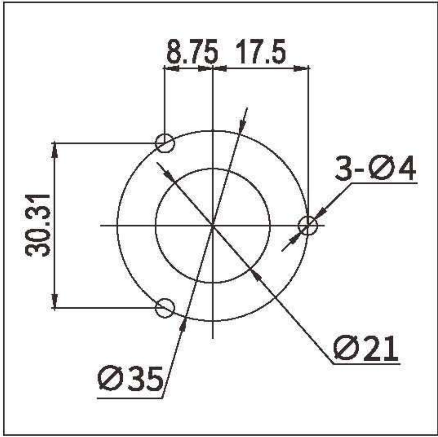
面板开孔尺寸
