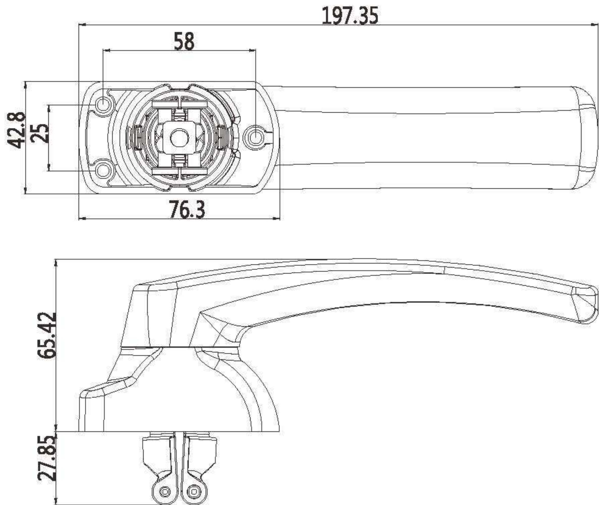
把手尺寸
