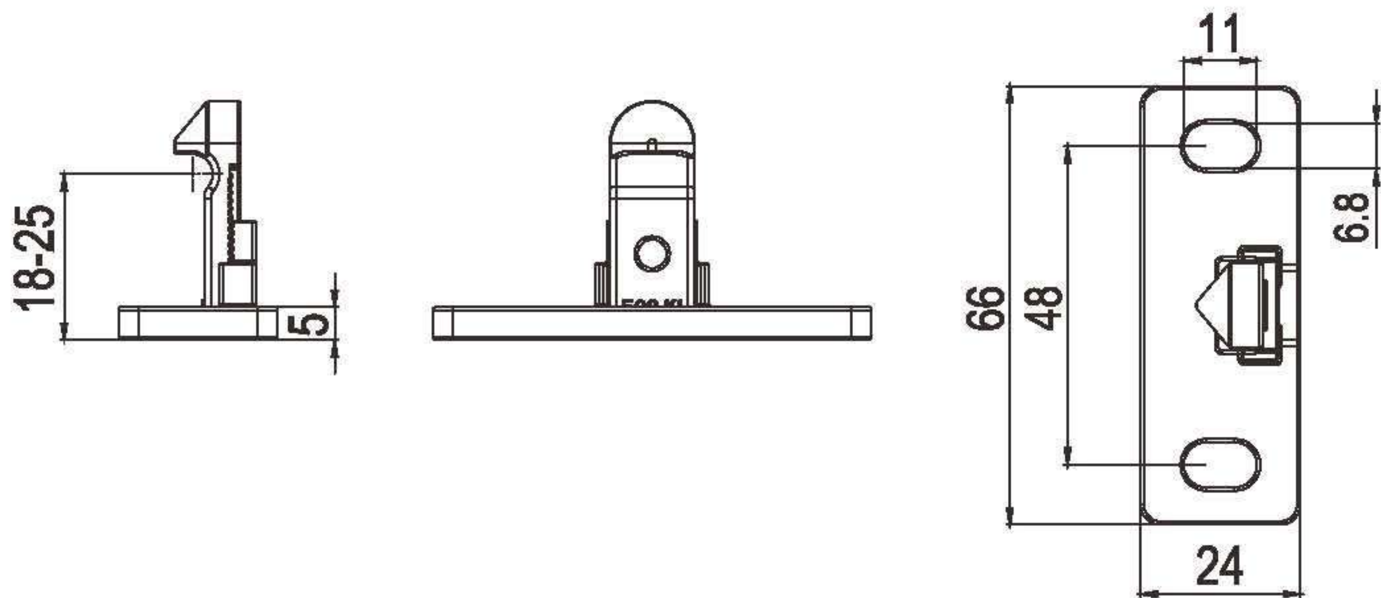
CH508 单级门扣
