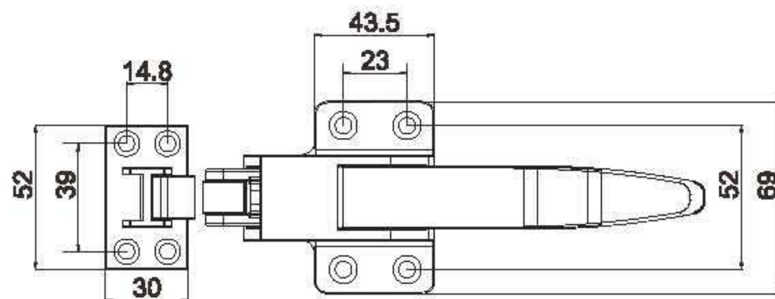
CH703-1 不锈钢
