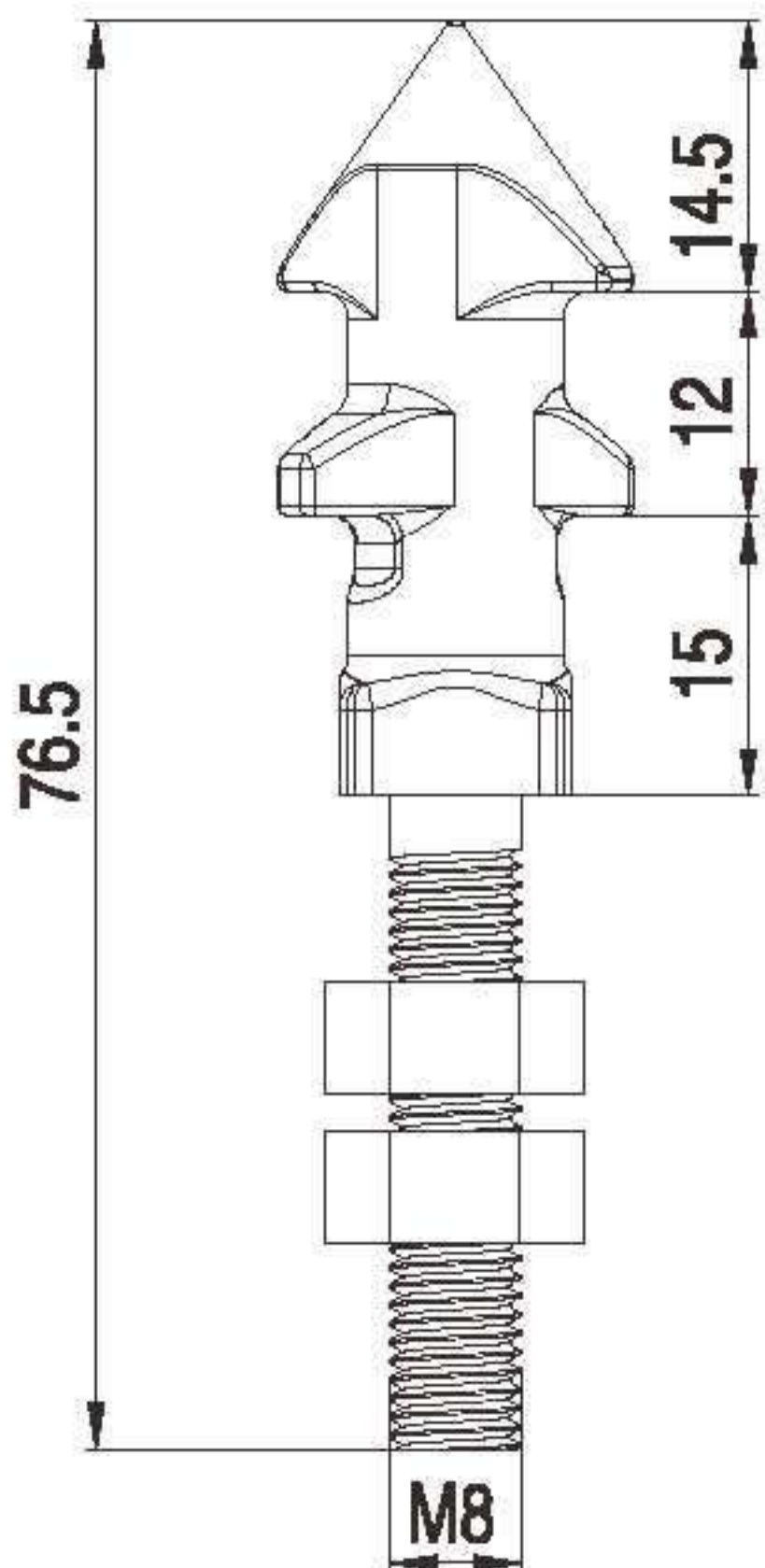
调节扣尺寸
