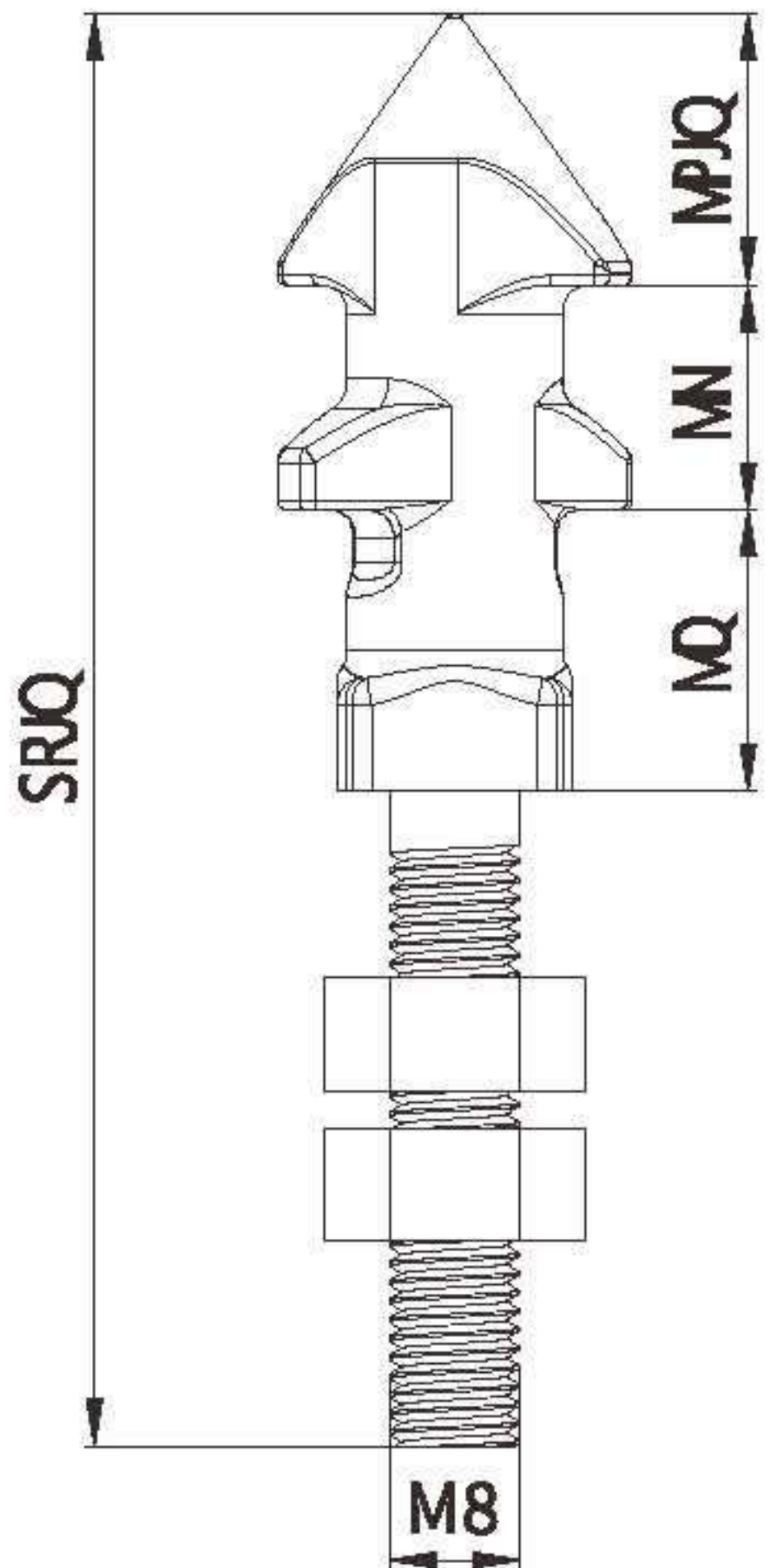
调节扣尺寸
