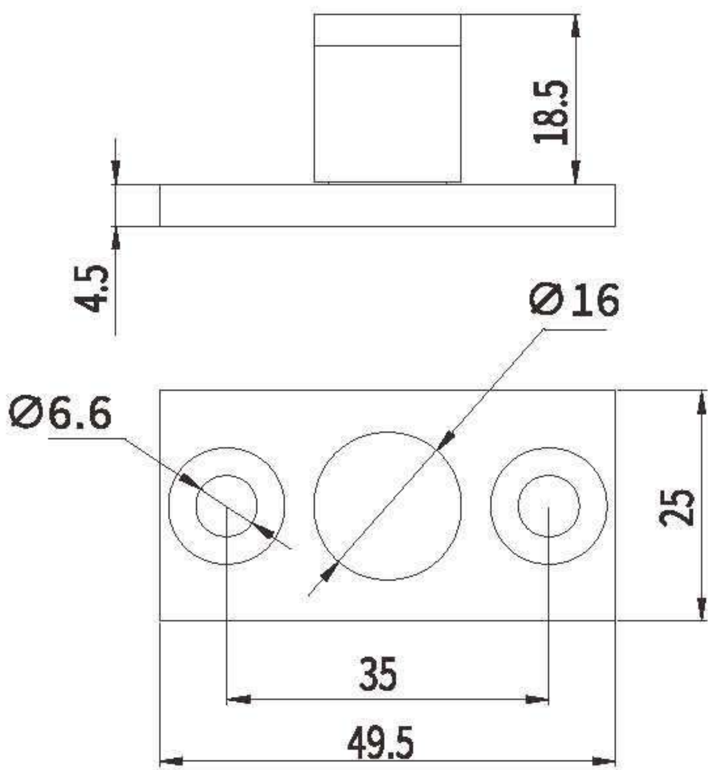
锁钩尺寸
