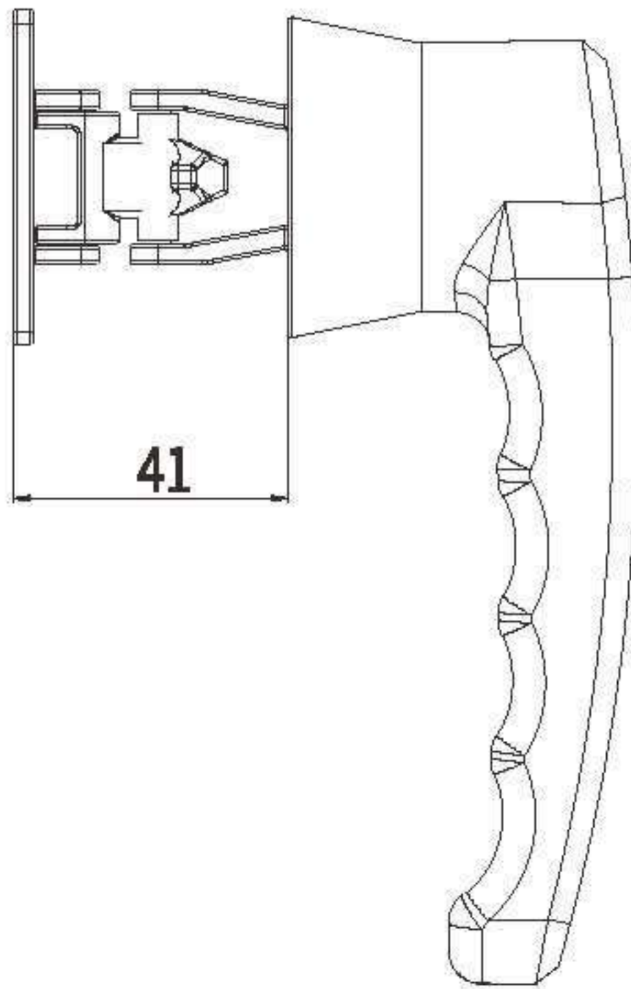
安装图
