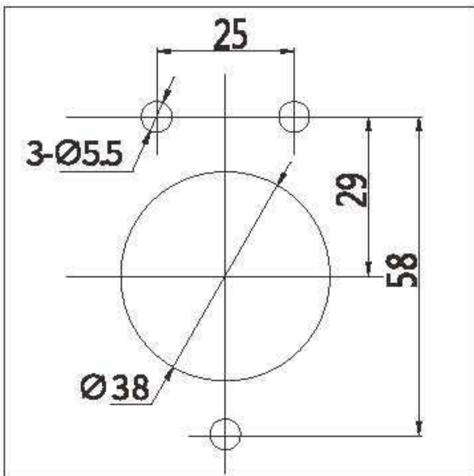
门板开孔尺寸
