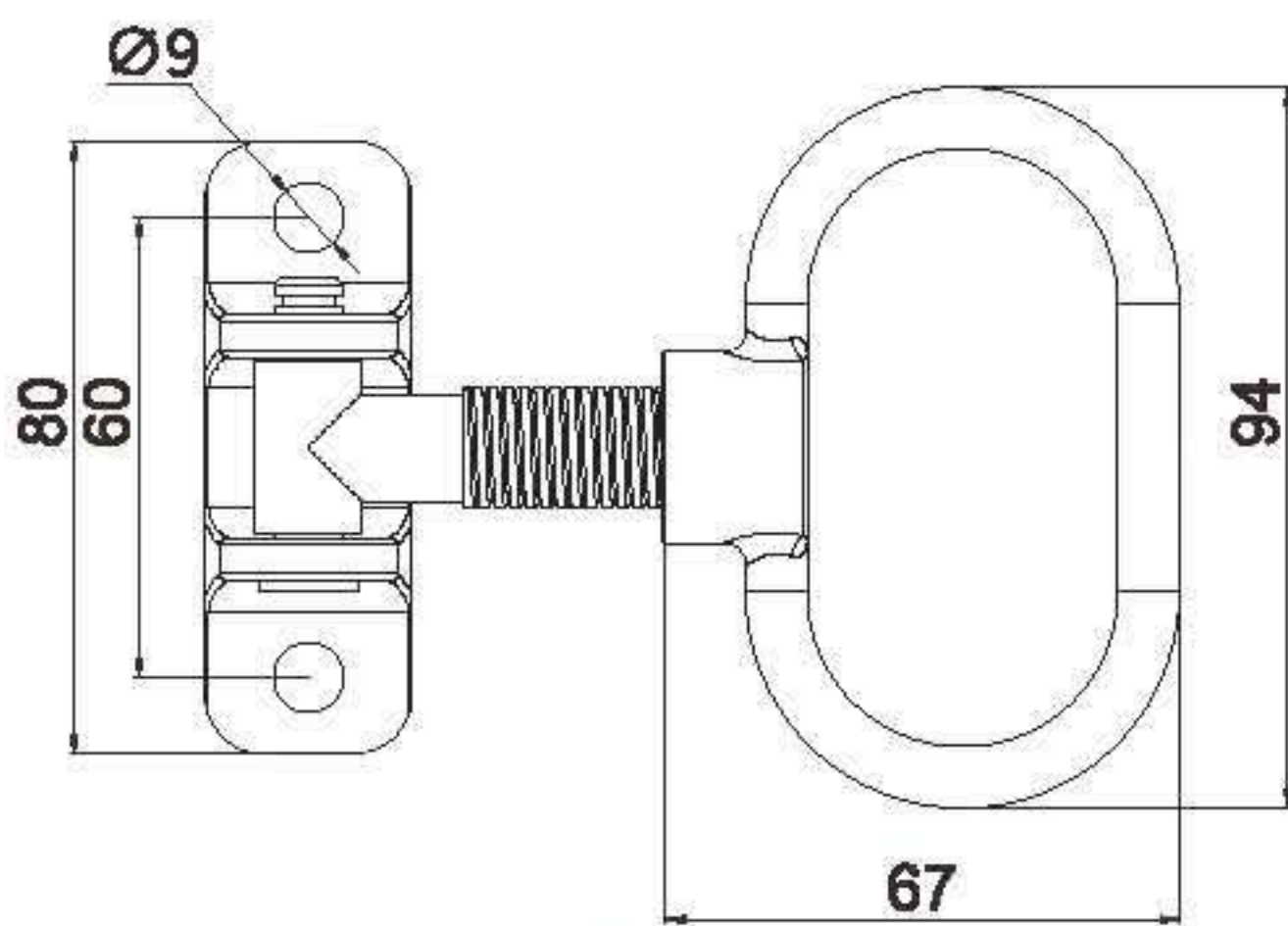
活动型 CH403-3
