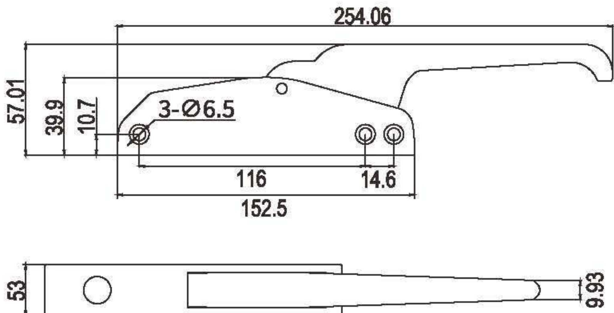
把手尺寸
