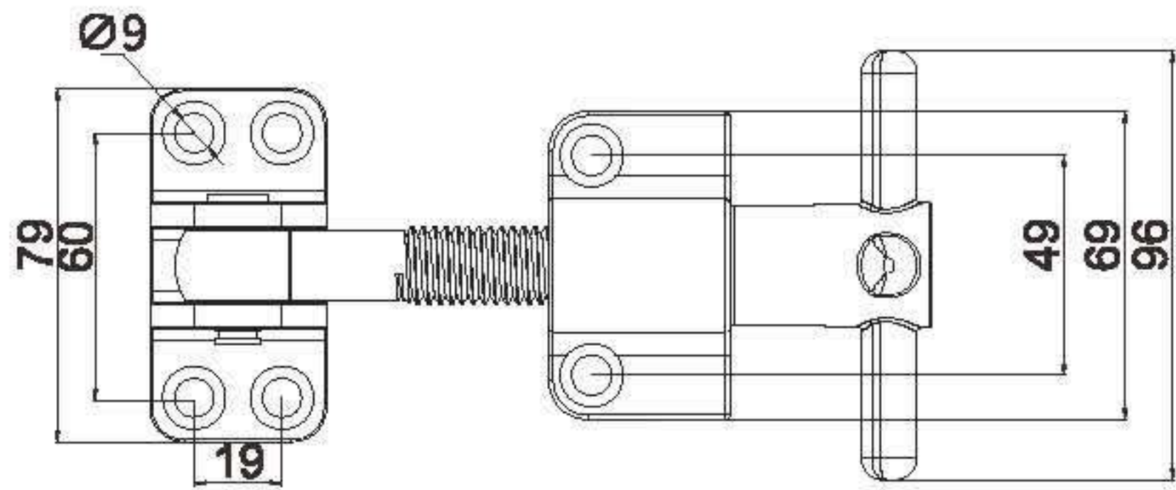
固定手轮 SY1-0405-2
