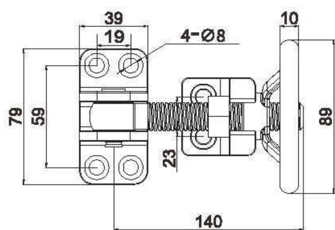
活动型 CH402-1
