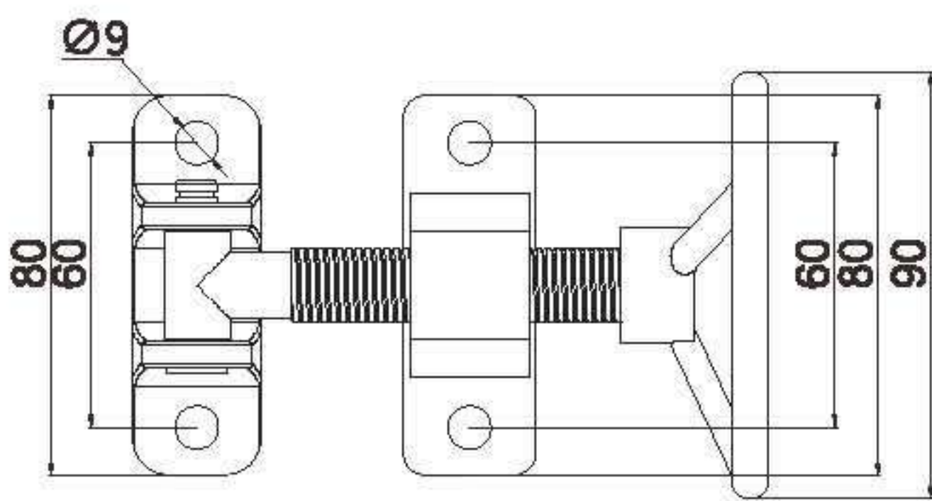
固定型 CH403-1
