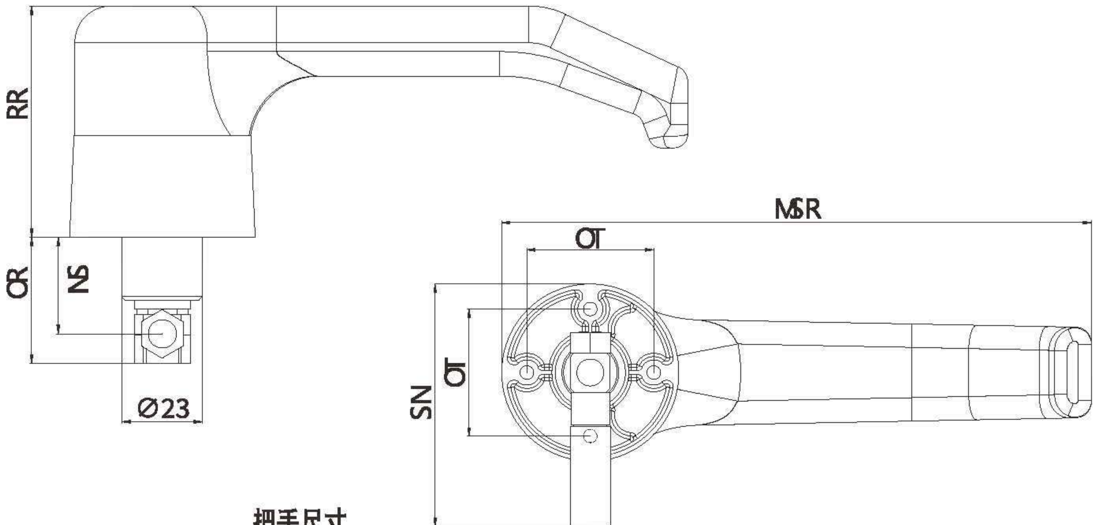
把手尺寸
