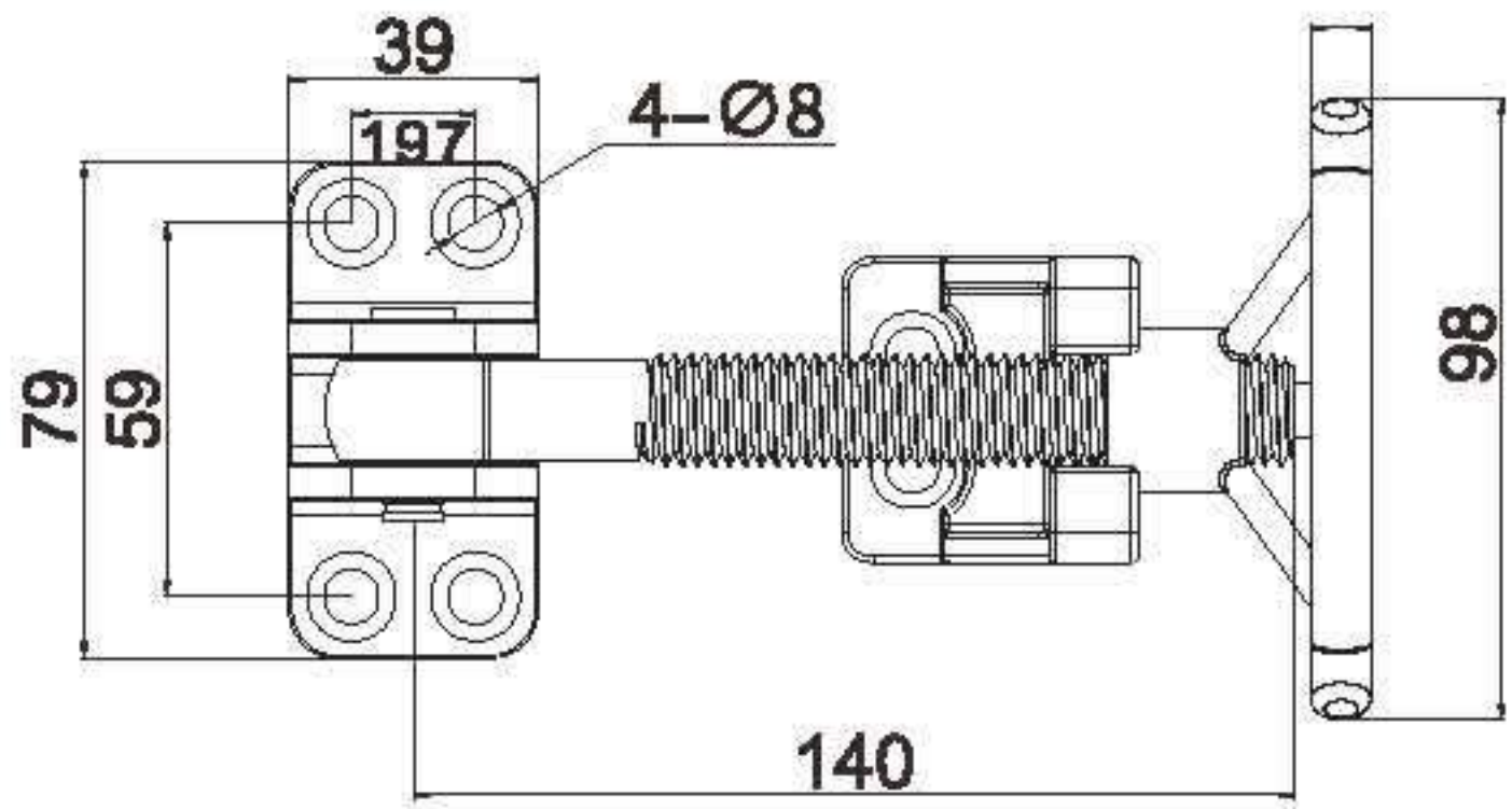
活动型 CH401-1
