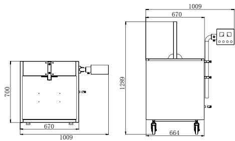
ST-6050 Hot Water Dip Tanks 热水收缩机
