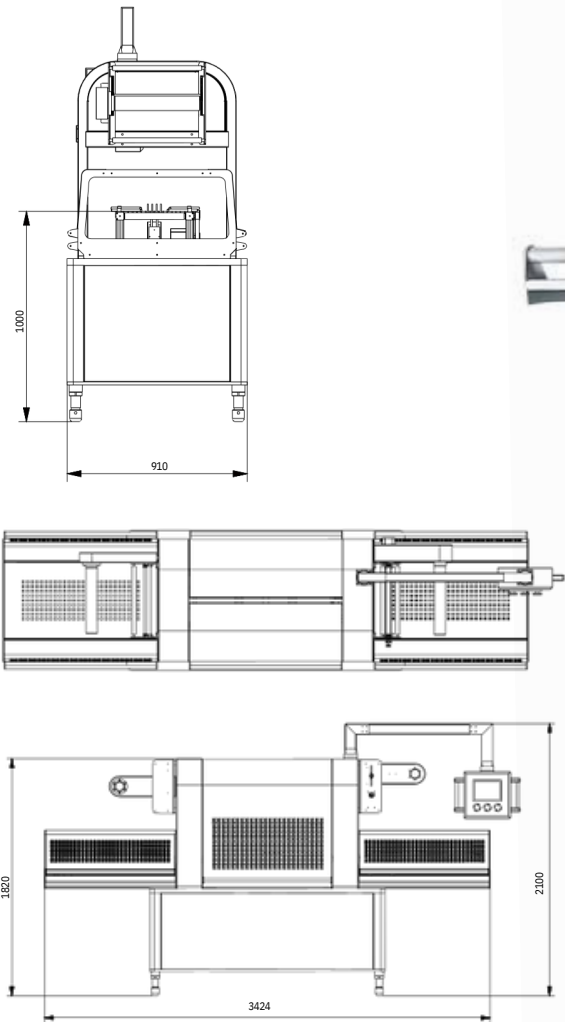
QT-700S Map Tray Sealer 气调封盒机
