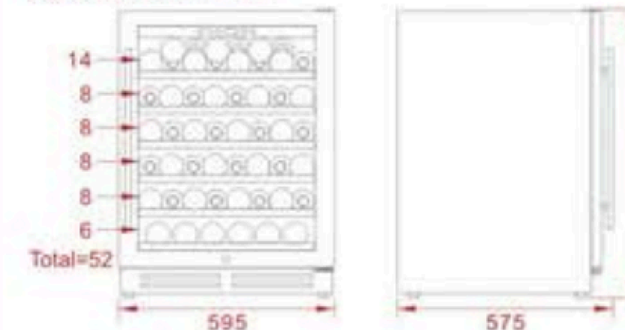
SRW-54S Product(W*D*H)mm
