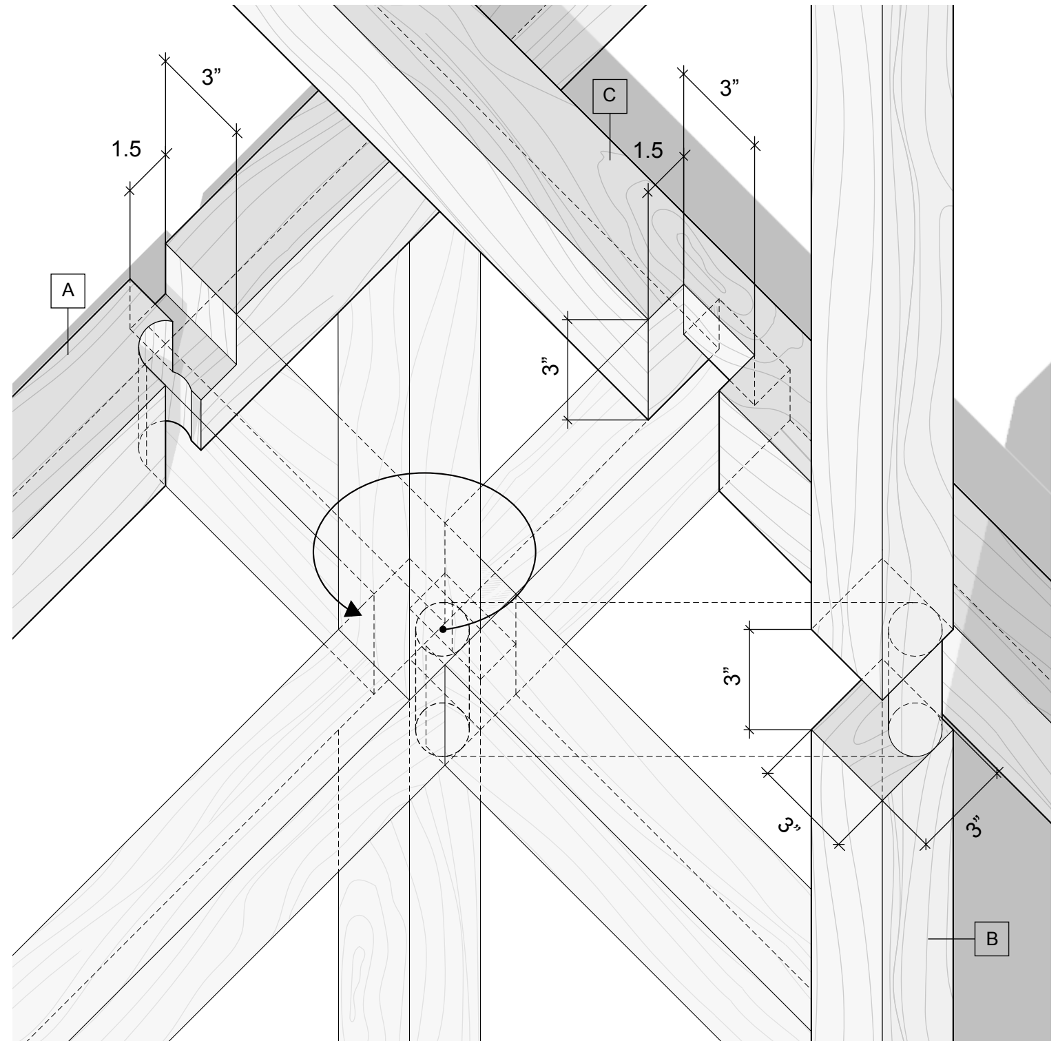
02. Sampo-gumi-shikuchi. Disassembled scale: 3'=1'=0"
