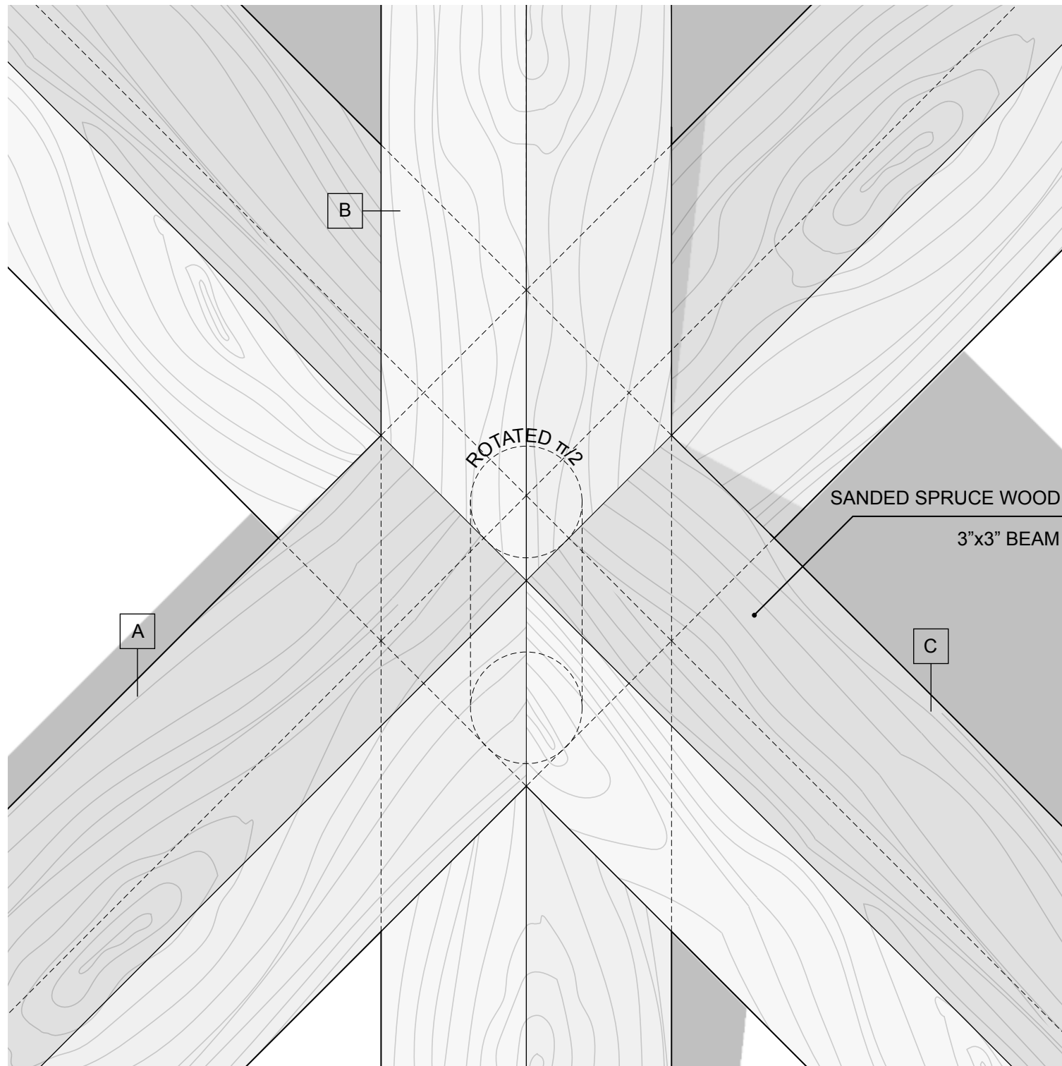
01. Sampo-gumi-shikuchi. Assembled scale: 1/2'=1'=0"
