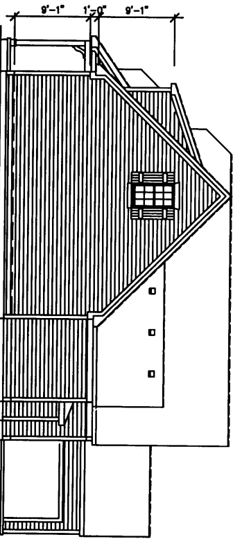
RIGHT ELEVATION
