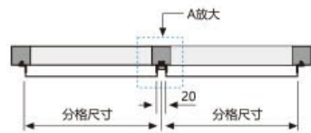
墙面铝单板安装示意图 镶条（明缝）式安装
