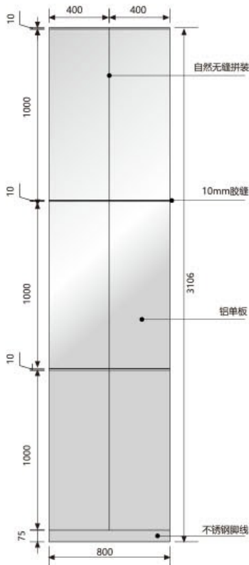
方柱子立面图(干挂式有缝)
