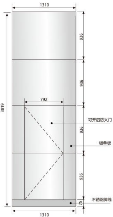
圆柱子立面图(无缝)
