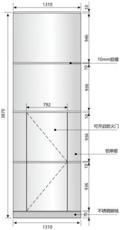
圆形柱子立面图(干挂式)
