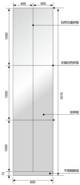
方柱子立面图(无缝)
