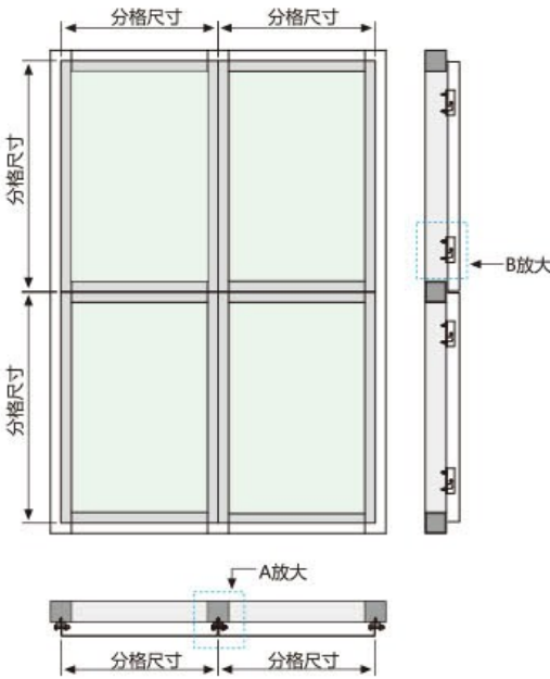
墙面铝单板安装示意图 （干挂式自然无缝拼装）式安装
