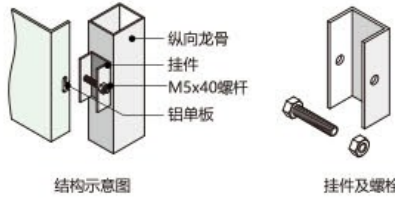
结构示意图
