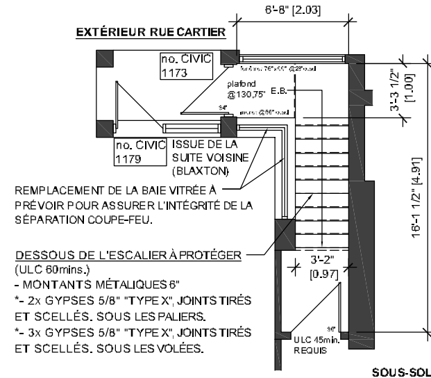
PLAN ISSUE 1 ECHELLE : 1/8"=1'-0"
