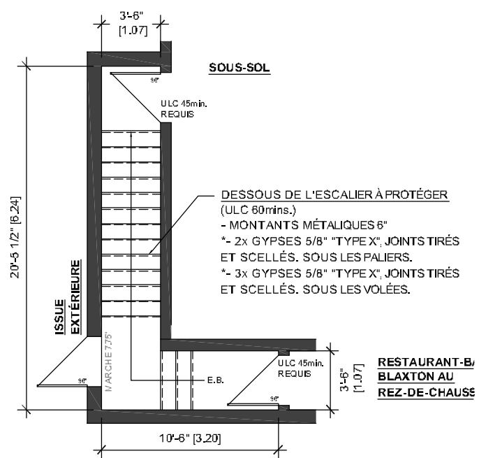
PLAN ISSUE 2 ECHELLE : 1/8"=1'-0"
