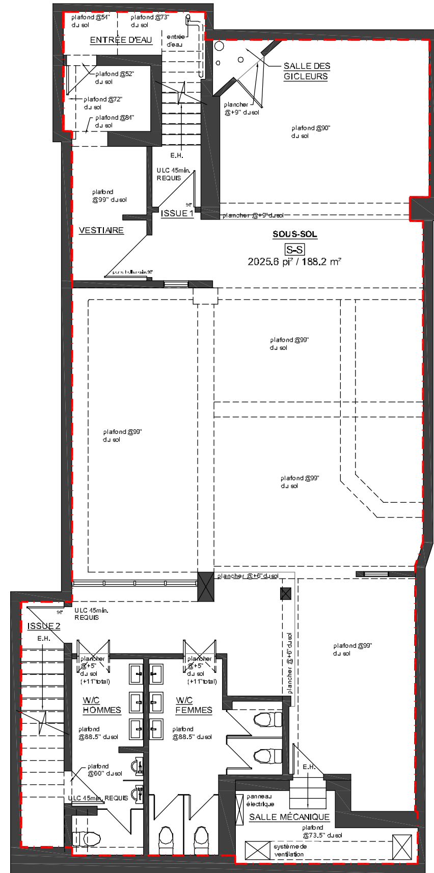
PLAN DE SOUS-SOL ECHELLE : 1/8"=1'-0"
