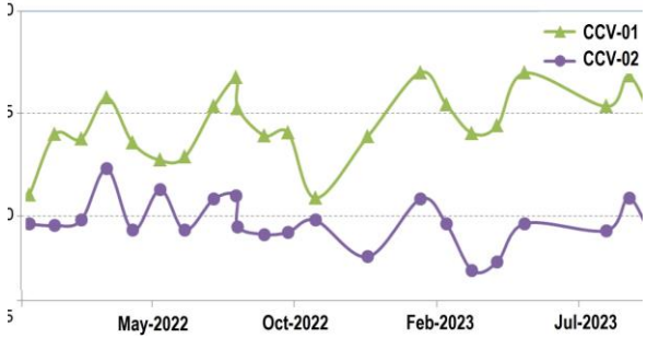
INSTALACIÓN y MONITOREO: PIEZOMETROS HIDRÁULICOS / CUERDA VIBRANTE
