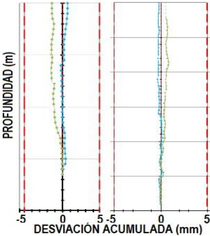
INSTALACIÓN y MONITOREO DE INCLINÓMETROS (ASTM D4429)
