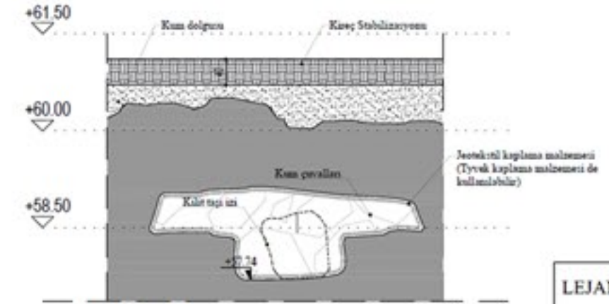
4-4 KESİTİ
