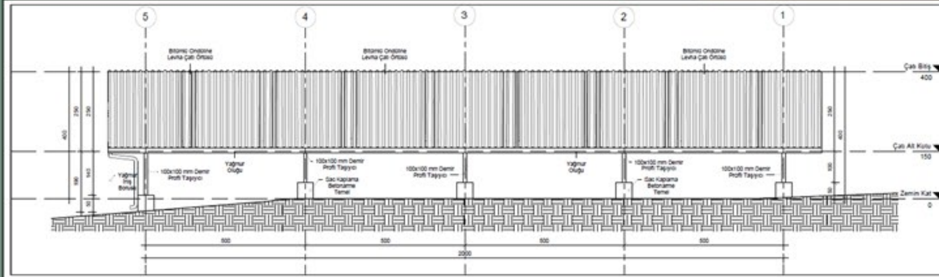
KUZİY CEPHESİ
