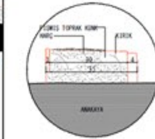
GÖRÜNÜŞ Ö:1/20
