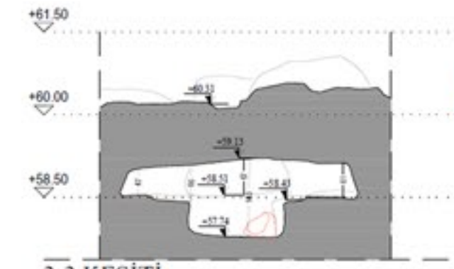
3-3 KESİTİ
