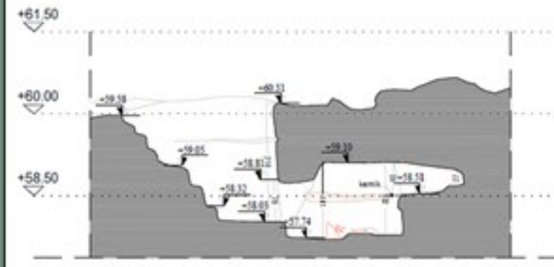
1-1 KESİTİ
