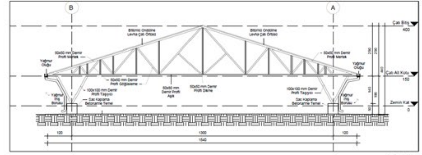
DOĞU CEPHESİ
