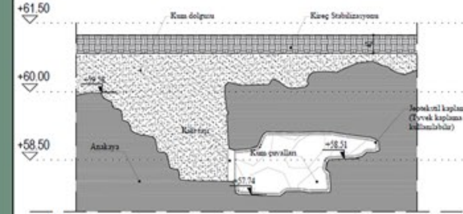
1-1 KESİTİ
