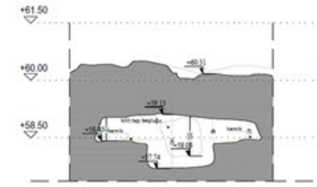
4-4 KESİTİ
