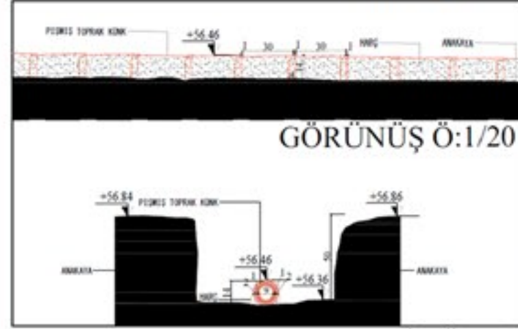
KESİT Ö:1/20
