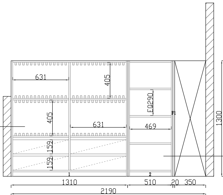
ELEVATION A
