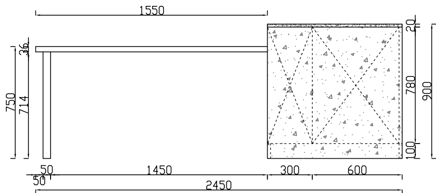
ELEVATION E
