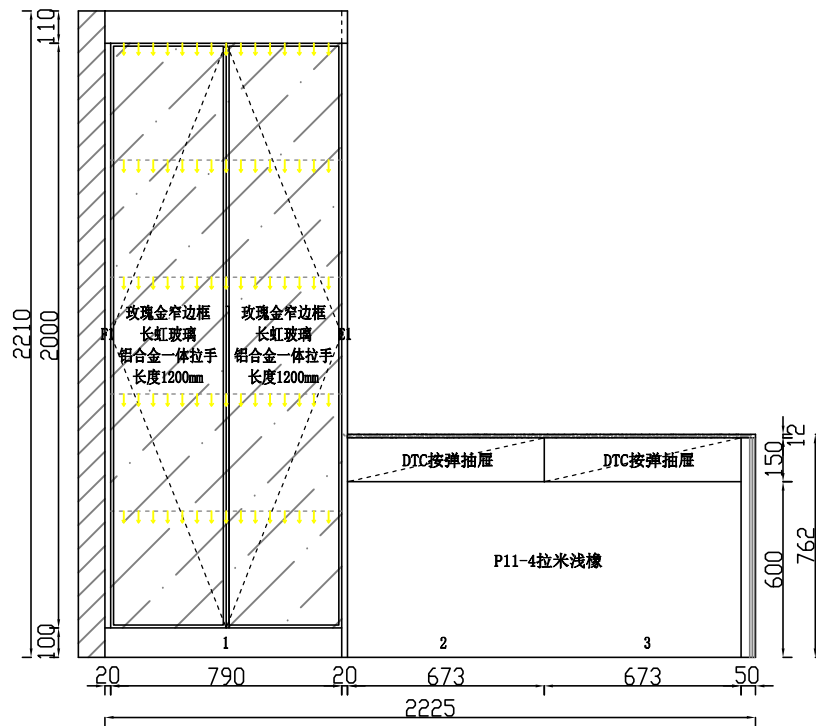
ELEVATION A
