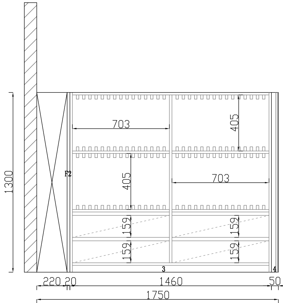
ELEVATION B
