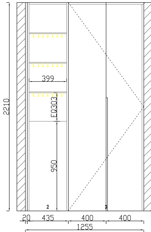
ELEVATION B
