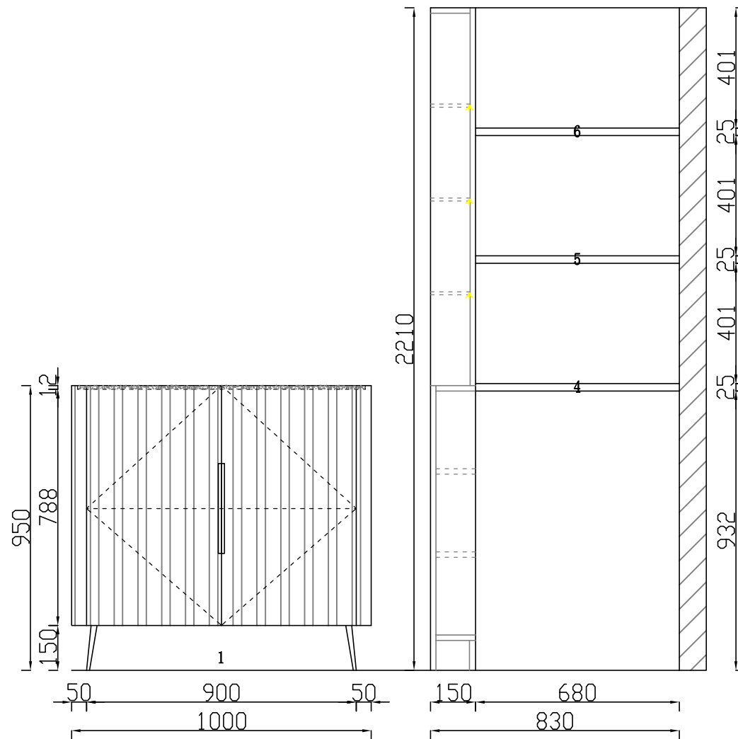
ELEVATION A
