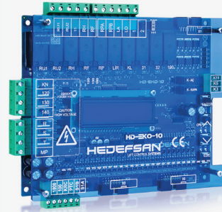
HEDEFSAN HD EKO 10 KONTROL KARTI [HEDEFSAN HD EKO 10 CONTROL CARD]
