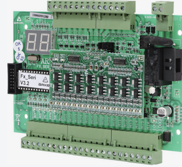
ARKEL FX-SERİ [ARKEL FX-SERIES]
