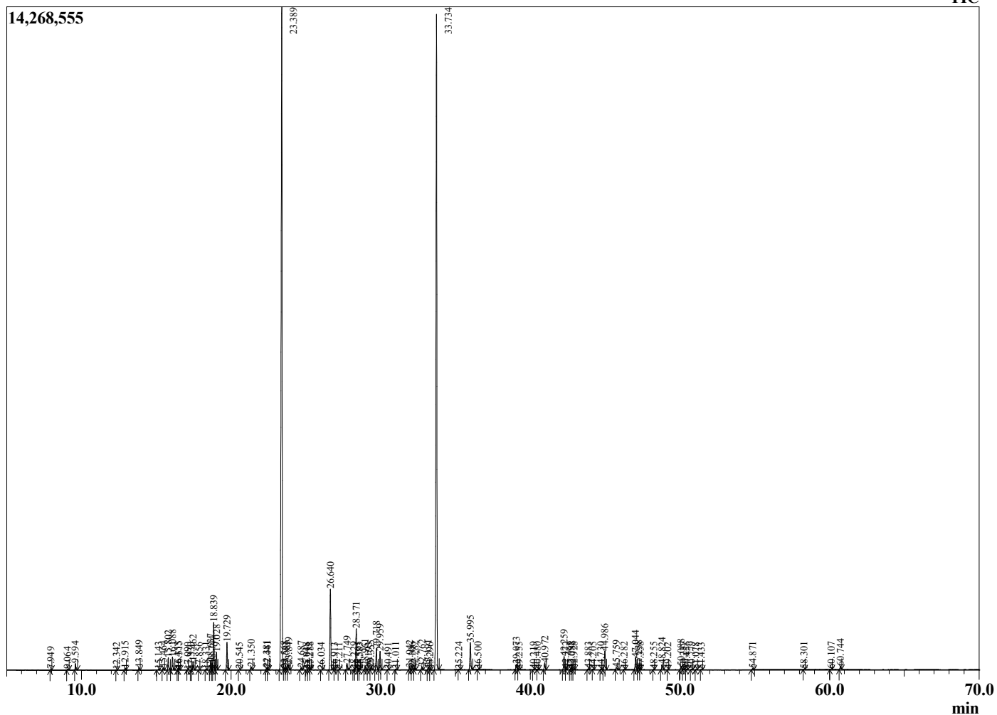
Chromatogram Lavandin Super-ESENCIA 1116
