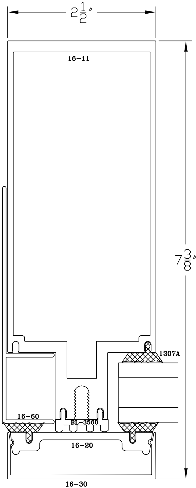
⑦ JAMB
