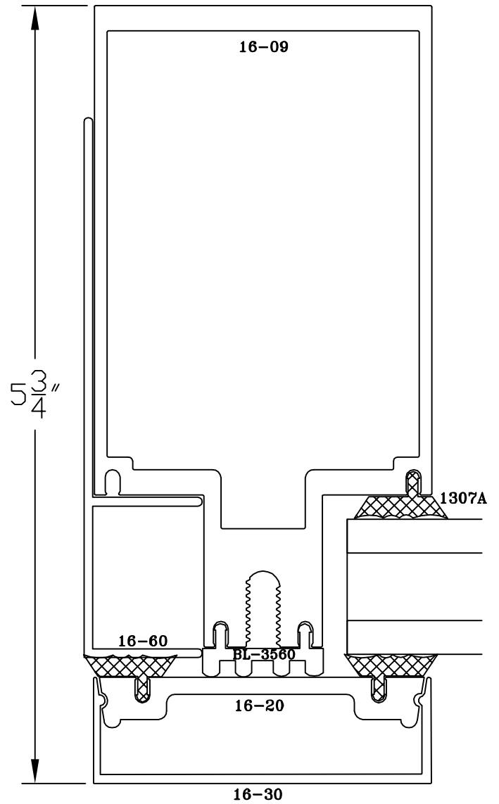
⑦A JAMB
