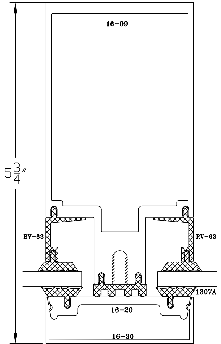
9A VERTICAL
