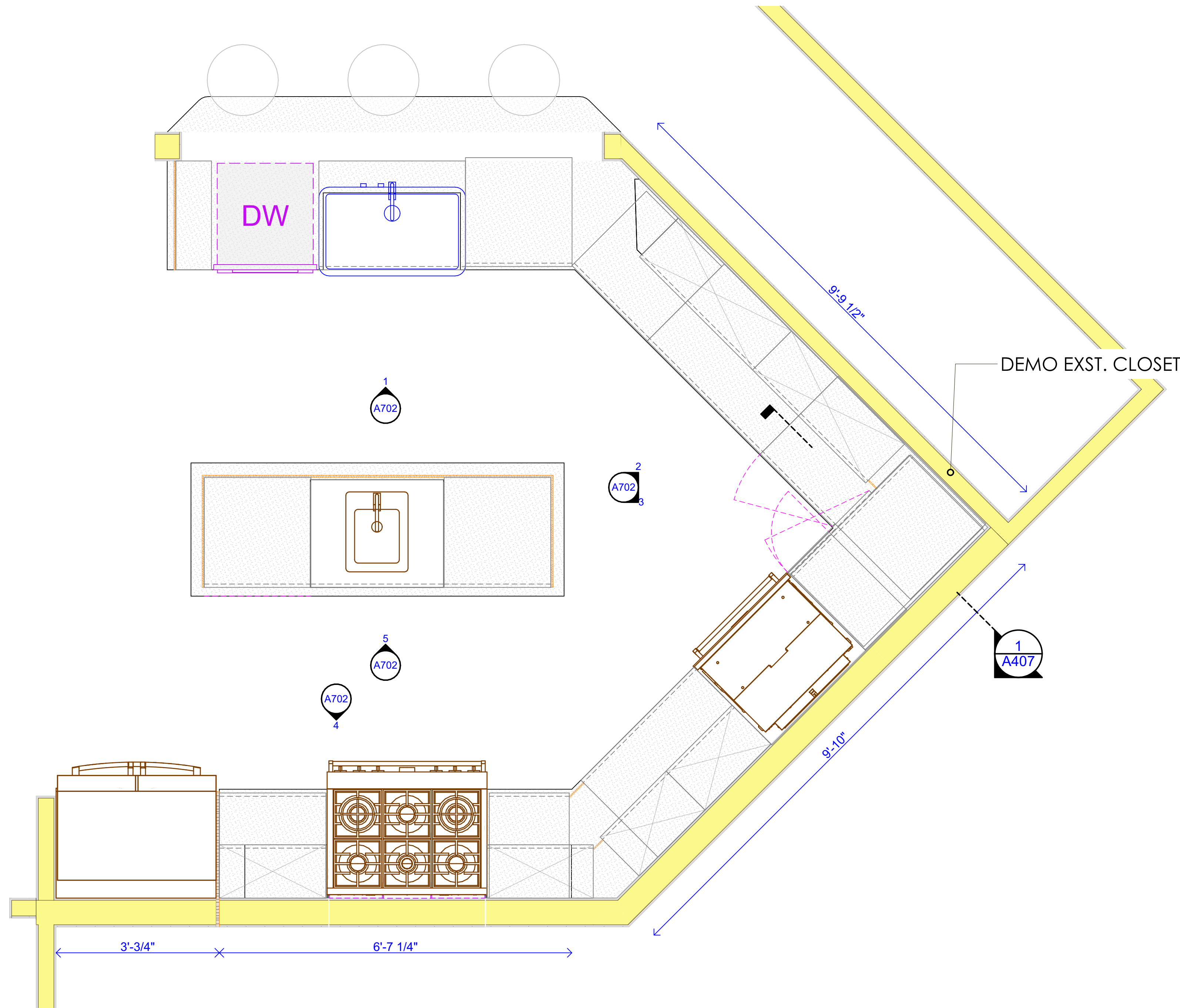
1. Level 1 SCALE: 3/4" = 1'-0"
