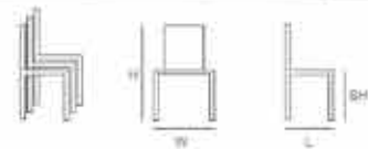
Item#: NET-05 Size: L50×W55×H83 SH:45cm
