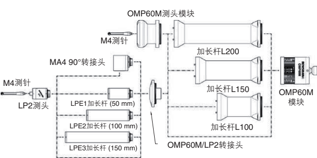
OMP60M / RMP60M模块化系统
