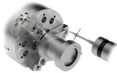
在车削中心上对已加工工件进行序中测量
