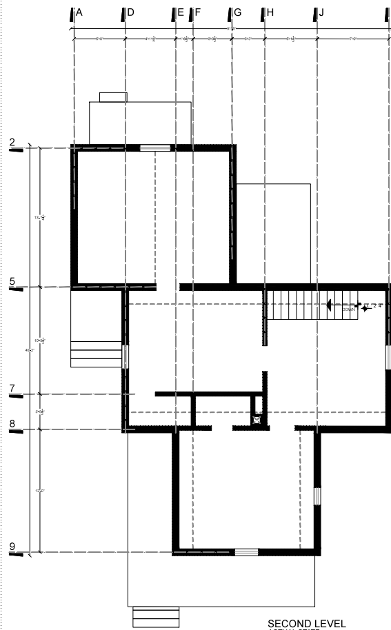
SECOND LEVEL ACTUAL STATE
