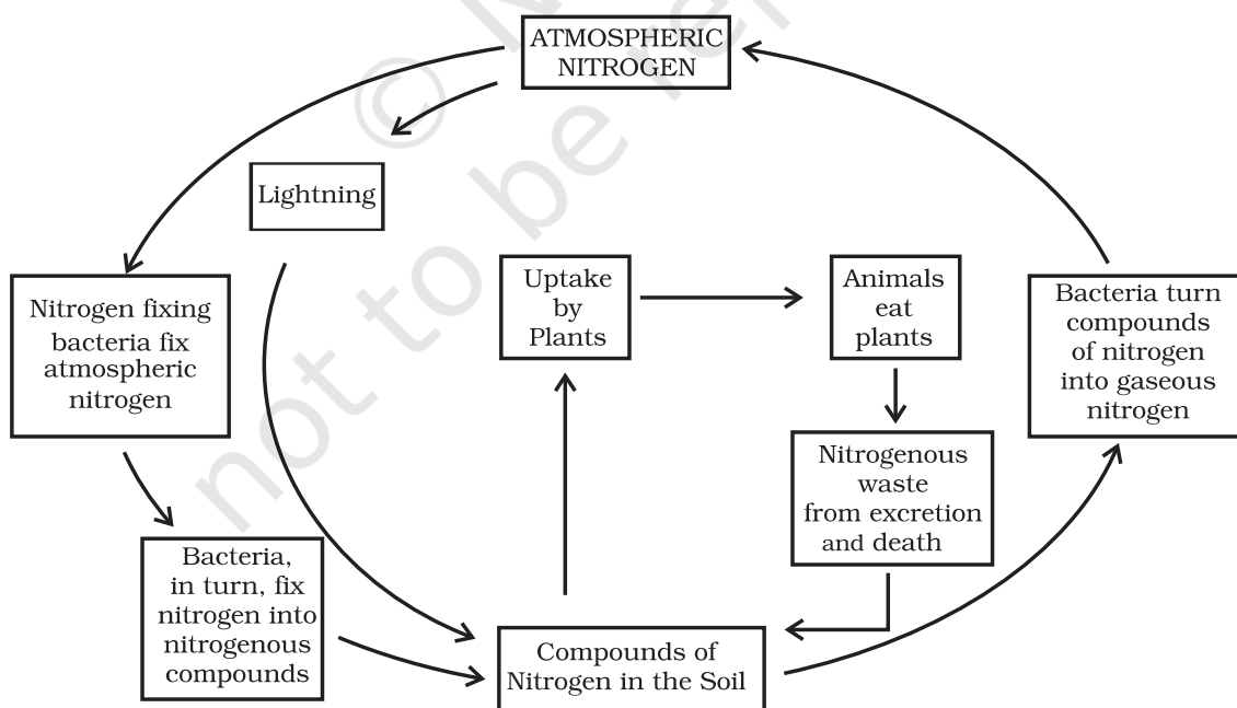
Fig. 2.10 : Nitrogen cycle
