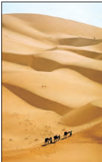
Fig. 3.9: Sand Dunes
