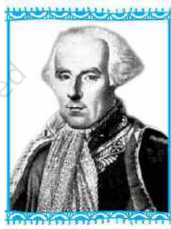
P.S. Laplace (1749-1827)
