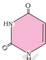
Uracil (Pyrimidine)
