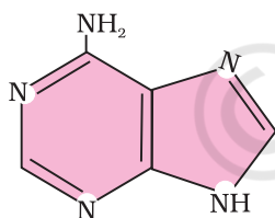
Adenine (Purine)
