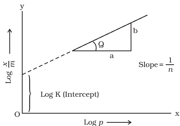
Fig. 5.2: Freundlich isotherm
