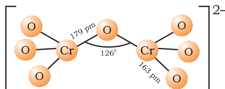
Dichromate ion
