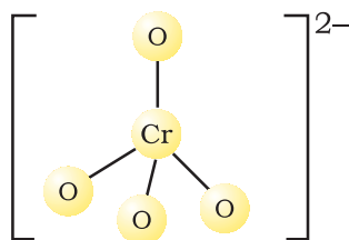
Chromate ion
