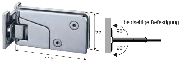
GTR-2001-90 zur beidseitigen Wandmontage, je 90° drehbar
