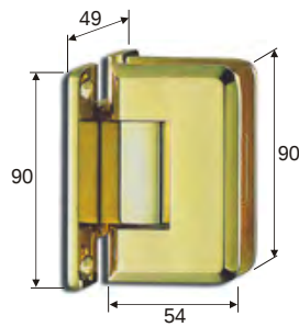
PIN037 & GTR zur beidseitigen Wandmontage, je 90° drehbar
