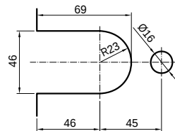
GTR-1002-180 Glas an Glas Befestigung Zur Montage eines Türflügels an ein feststehendes Glasteil im 180° Winkel
