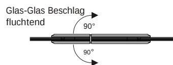
PIN180 & GTR Glas an Glas, je 90° drehbar PIN380 5° Feinjustierung
