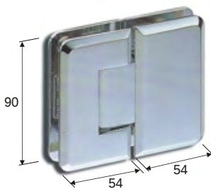
PIN180 & GTR Glas an Glas, je 90° drehbar PIN380 5° Feinjustierung
