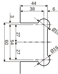
SDH037 zur beidseitigen Wandmontage, je 90° drehbar
