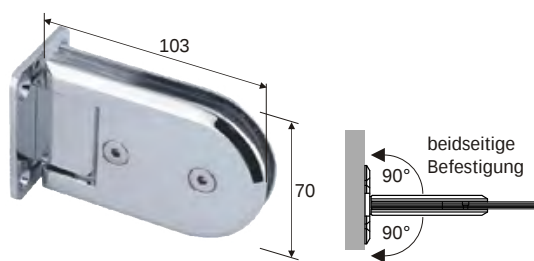
GTR-301-90 zur beidseitigen Wandmontage, je 90° drehbar
