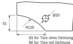
GTR-2001-90 zur beidseitigen Wandmontage, je 90° drehbar
