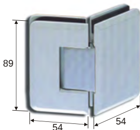
PIN045 & GTR Glas an Glas, mit Feststellung bei 135° PIN345 Feinjustierung
