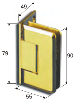
PIN044 & GTR zur einseitigen Wandmontage, je 90° drehbar
