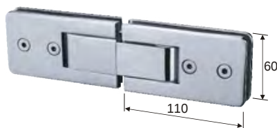
GTR-1002-180 Glas an Glas Befestigung Zur Montage eines Türflügels an ein feststehendes Glasteil im 180° Winkel
