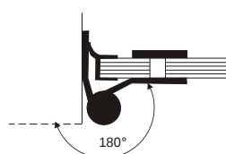
GTR-05 Wandbefestigung
