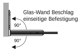
PIN044 & GTR zur einseitigen Wandmontage, je 90° drehbar
