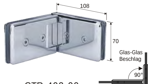
GTR-402-90 Glas an Glas, zur Montage eines Türflügels an einem feststehenden Seitenteil 90°, je 90° drehbar
