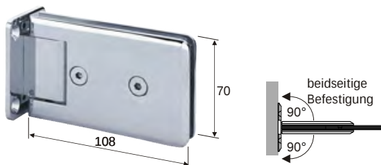
GTR-401-90 zur beidseitigen Wandmontage, je 90° drehbar
