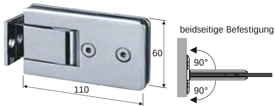
GTR-1001-90 zur beidseitigen Wandmontage, je 90° drehbar
